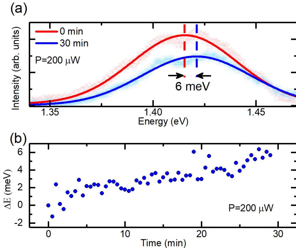
Figure 5: (a) Spectres photoluminescence de l'exciton inter-couche au début et à la fin de l'exposition à un laser haute puissance. (b) Evolution temporelle de l'énergie de l'exciton inter-couche photoluminescence à haute puissance d'excitation.
