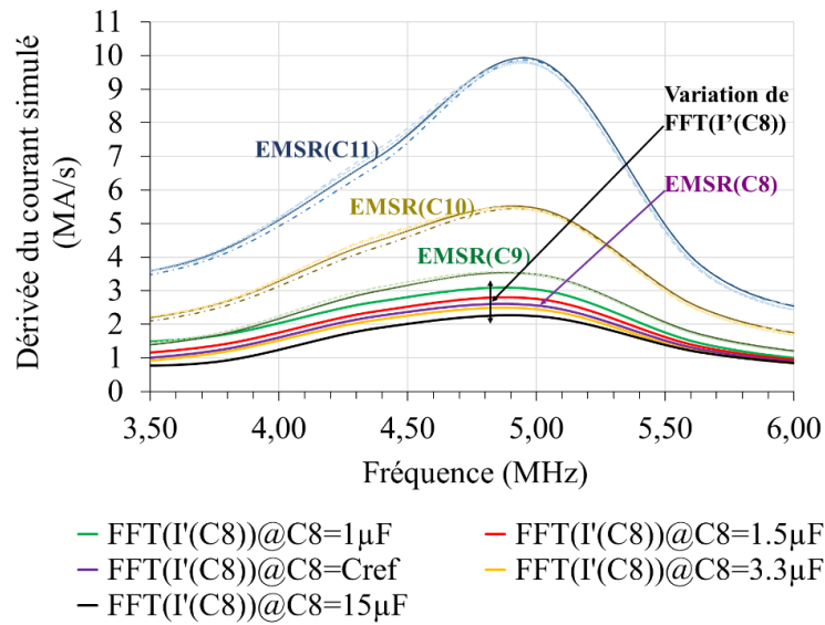
Figure 4. 36. FFT des dérivées de courant simulé dans les condensateurs de découplage lorsque C8 prend plusieurs valeurs (C8=1µF, C8=1.5µF, C8=Cref=2.2µF, C8=3.3µF, C8=15µF)
