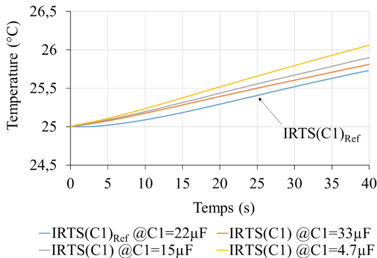
Figure 5. 11. Comparaison des signatures thermiques infrarouges du condensateur C1 pour trois valeurs erronées ( C1=4.7\mu F , C1= 15\mu F , C1= 33\mu F ) par rapport à sa signature de référence \text{IRTS}(C1)_{Ref} .
