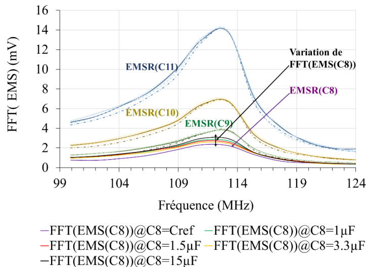
Figure 4. 37. FFT des EMS mesurés au-dessus des condensateurs de découplage lorsque C8 prend plusieurs valeurs (C8=1µF, C8=1.5µF, C8=Cref=2.2µF, C8=3.3µF, C8=15µF)
