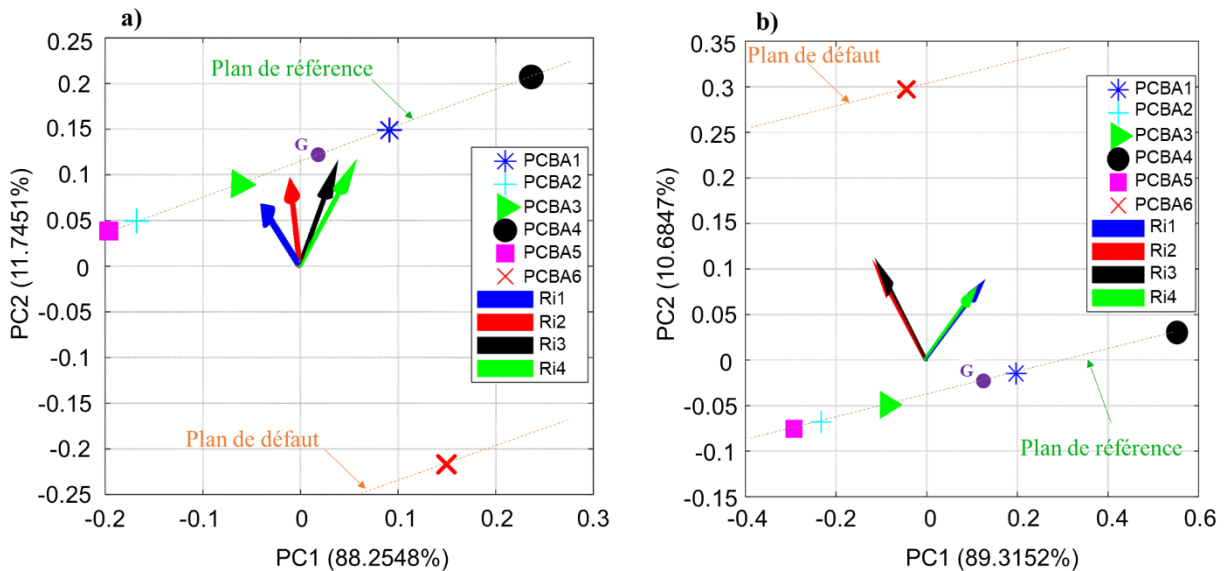
Figure 5. 24. Résultats d'analyse PCA pour 6 PCBA avec PCBA6 défectueux : a) cas\ j : tous les condensateurs ont des valeurs erronées supérieures à C_{ref} b) cas\ f : tous les condensateurs ont des valeurs erronées inférieures à C_{ref}
