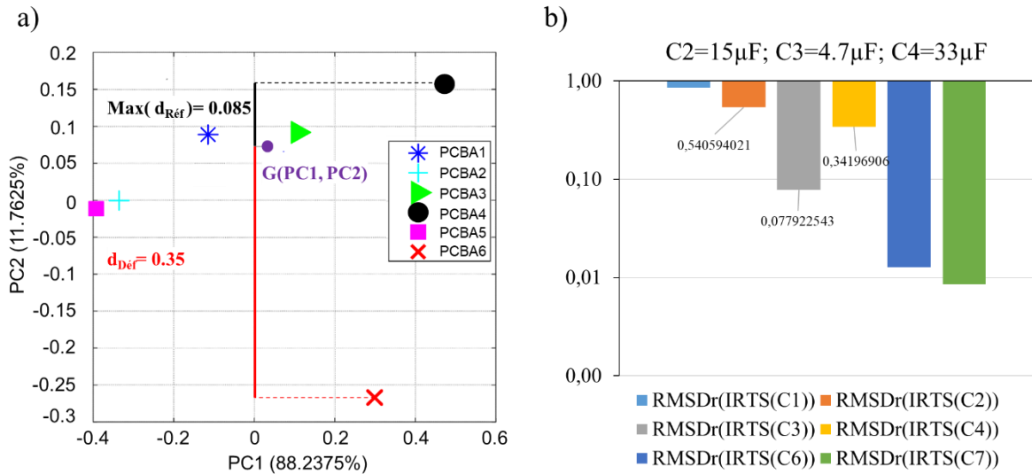
Figure 5. 18. a). Résultats de l'analyse PCA pour 6 PCBA avec un PCBA défectueux : PCBA6 contenant 3 condensateurs de valeurs erronées ( C2=15\mu F , C3=4.7\mu F et C4=33\mu F ); b) comparaison des RMSD_r pour ce cas de défauts
