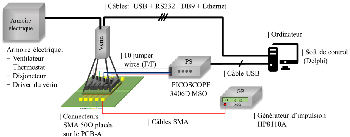
Figure 6. 16. Banc de test du prototype ACR-P
