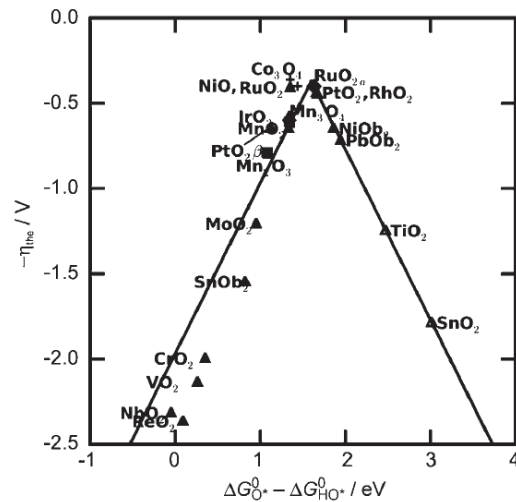
Figure I.27 : Courbe volcan représentant la surtension en fonction de la différence d'enthalpie libre associée aux intermédiaires de réaction formés pendant l'OER pour plusieurs catalyseurs[109]
