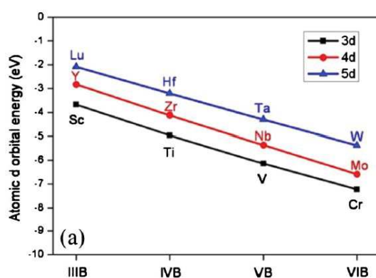
Figure I.25 : Énergie des orbitales d de plusieurs métaux de transitions[97]
