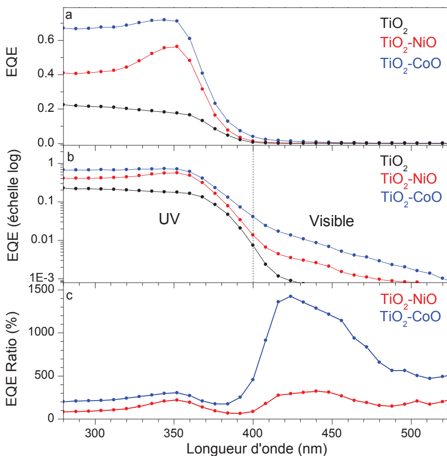
Figure IV.20 : Courbes d'EQE des nanotubes de \text{TiO}_2 avant et après décoration avec des nanoparticules de CoO et NiO en (a) échelle linéaire, (b) échelle logarithmique et (c) ratio d'EQE décrit selon l'équation IV.18
