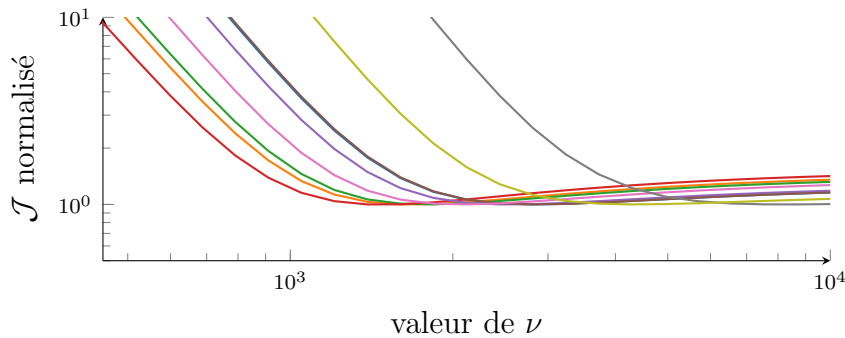
FIGURE 4 – Évolution du coût fatigues \mathcal{J} avec le paramètre de la MPC quadratique \nu pour 9 vents différents, normalisé par le minimum de fatigue obtenu pour chaque vent, chaque couleur représentant une réalisation du vent.
