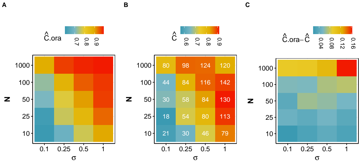
FIGURE 2.9 – C-index médians oracles (A) et estimés (B), et différences médianes entre les C-index oracles et estimés (C) pour différents paramètres de simulation pour LGG et la pénalisation elastic net - données simulées.
