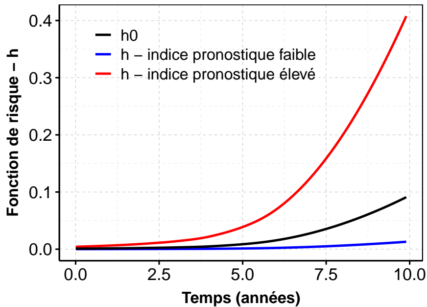
FIGURE 1.5 – Fonction de risque pour différents patients.
