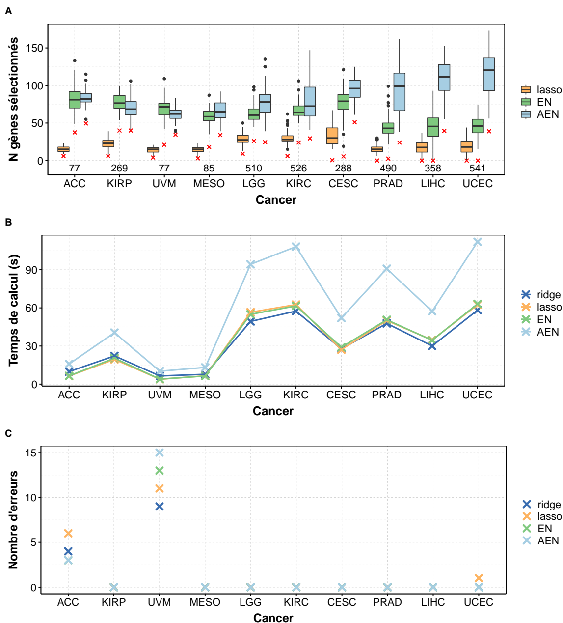
FIGURE 2.4 – Nombre de gènes sélectionnés (A), temps de calcul médian (s) (B), et nombre d'erreurs dans le calcul du C-index avec \lambda_{\min} (C) des méthodes de pénalisation obtenus avec les données mRNA-seq.
