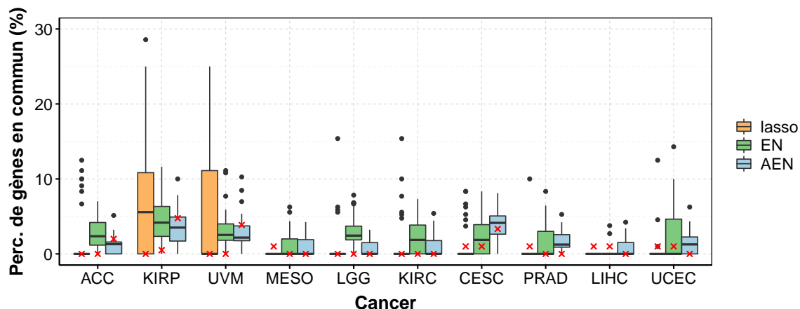
FIGURE 2.14 – Stabilité des gènes sélectionnés.
