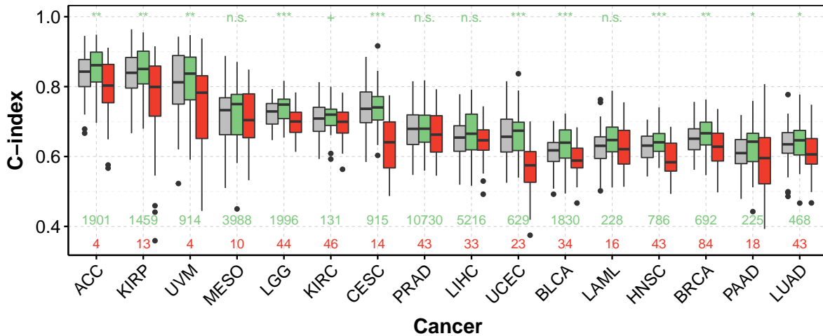
FIGURE 3.7 – C-index obtenus sans pré-filtrage (gris), avec le pré-filtrage bi-dimensionnel et la pénalisation elastic net (vert), et avec l'algorithme Sure Independence Screening (rouge) pour les 16 cancers de TCGA étudiés.
