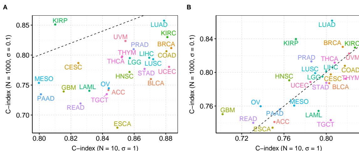
FIGURE 2.11 – C-index médians obtenus avec elastic net (A) et ridge (B) pour différents paramètres de simulations contenant la même quantité d'information pour les 26 cancers de TCGA étudiés - données simulées.
