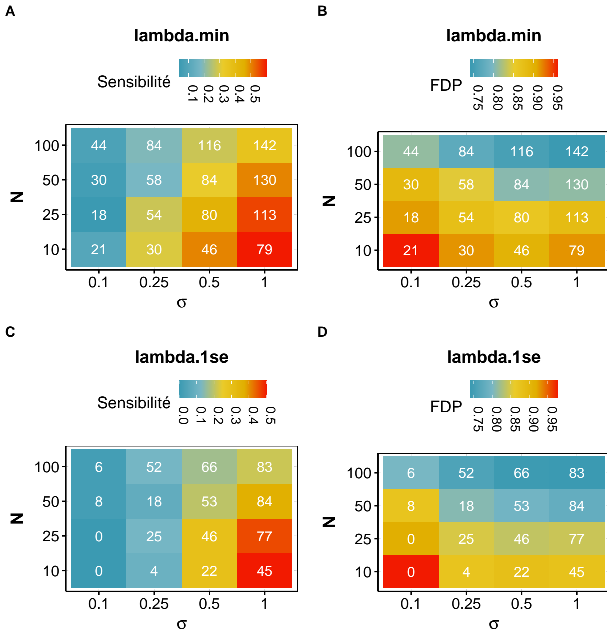
FIGURE 2.15 – Sensibilités (A, C) et taux de fausses découvertes (FDP) (B, D) obtenus avec \lambda_{min} (A, B) et \lambda_{1se} (C, D) pour LGG et la pénalisation elastic net - données simulées.
