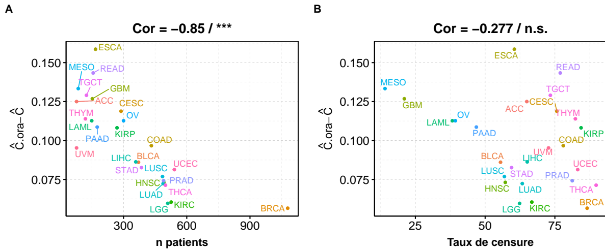
FIGURE 2.13 – Différences médianes entre les C-index oracles et estimés en fonction du nombre de patients (A) et du taux de censure (B) pour l'ensemble des 26 cancers étudiés.
