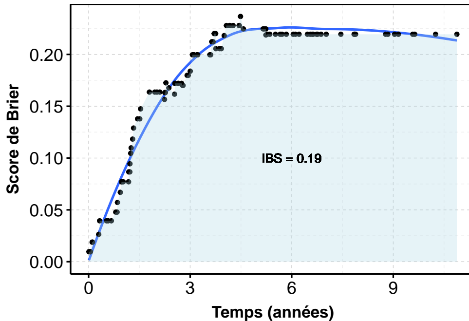
FIGURE 1.7 – Score de Brier en fonction du temps calculé avec les données d’expression d’ARN messagers de TCGA pour le cancer du rein à cellules claires (KIRC).
