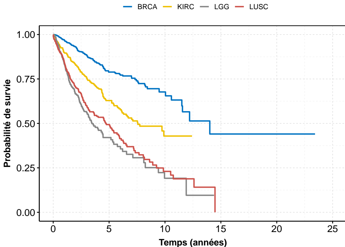
FIGURE 1.4 – Courbes de survie obtenue à partir des données TCGA pour quatre cancers. Selon les recommandations de LIU et collab. [2018b], la survie globale est utilisée pour KIRC et LUSC, et la survie sans récurrence est utilisée pour BRCA et LGG.
