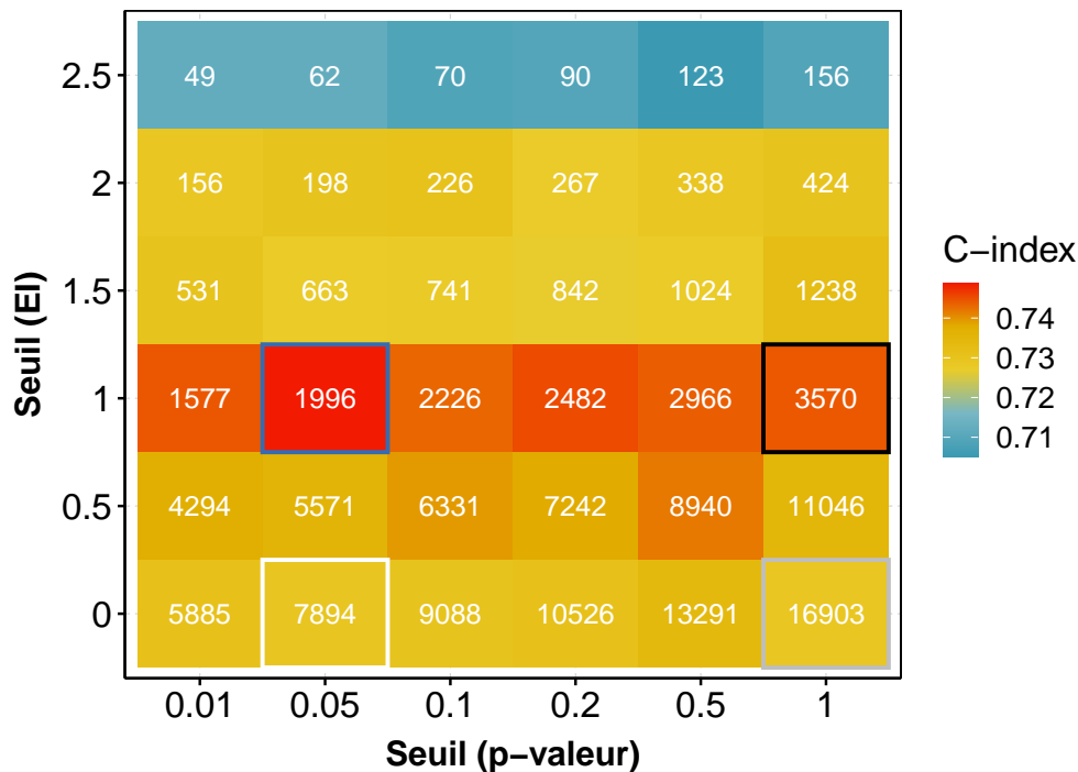
FIGURE 3.2 – C-index médians obtenus pour différents seuils de pré-filtrage pour LGG. Pour chaque seuil, les C-index sont calculés par 10 répétitions d'une validation croisée en K = 5 groupes, et le pré-filtrage des gènes est fait sur le jeu de données d'apprentissage. Dans chaque case, le chiffre indiqué en blanc correspond au nombre médian de gènes retenus après le pré-filtrage bi-dimensionnel. Case entourée de noire : résultats obtenus avec uniquement un pré-filtrage sur l'EI; case entourée de blanc : résultats obtenus avec uniquement un pré-filtrage sur la p-valeur du modèle de Cox univarié; case entourée de bleu : résultats obtenus dans le cas optimal ( i.e. C-index médian le plus important); case entourée de gris : résultats obtenus sans pré-filtrage.
