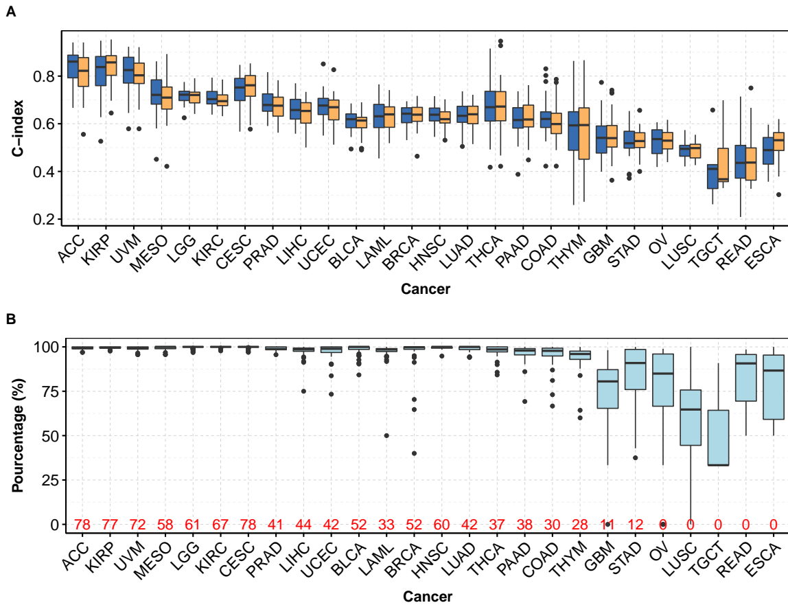
FIGURE 5.1 – C-index obtenus avec elastic net avec uniquement le niveau d’expression des gènes (bleu), et avec l’ajout des termes d’interactions (jaune) (A), et proportions de termes quadratiques sélectionnés.
