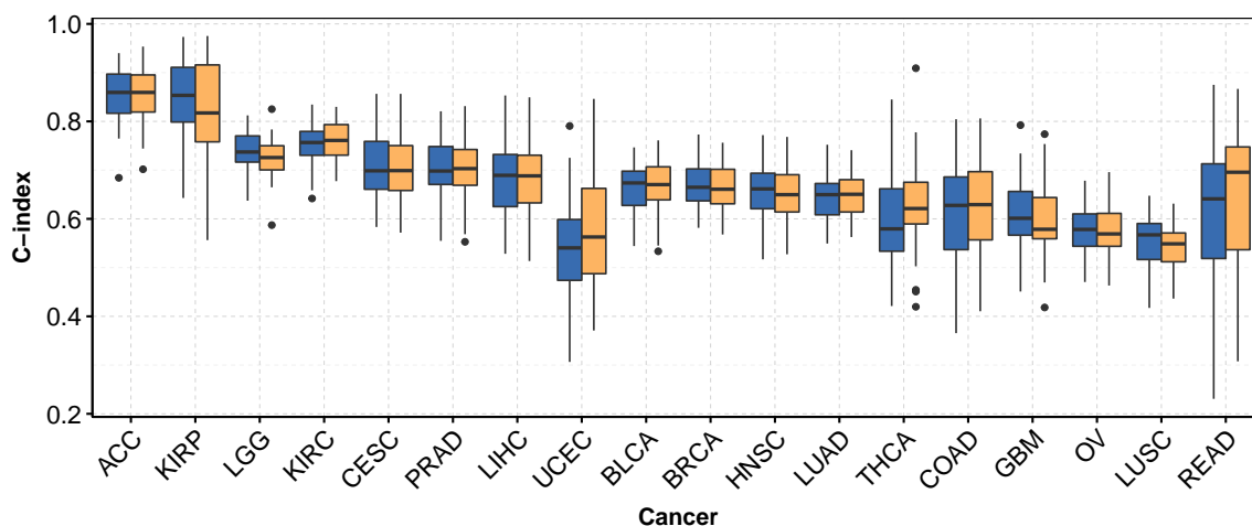
FIGURE 5.4 – C-index obtenus avec les variables cliniques et les indices pronostiques des données mRNA-seq (bleu), et avec les variables cliniques et les indices pronostiques des données mRNA-seq, xCell, et de pureté de la tumeur (jaune).
