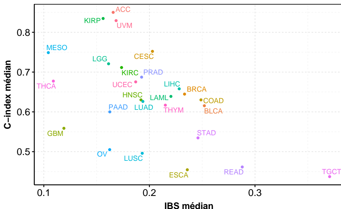
FIGURE 2.2 – C-index médians en fonction des IBS médians calculés avec la pénalisation elastic pour l'ensemble des 26 cancers de TCGA étudiés.
