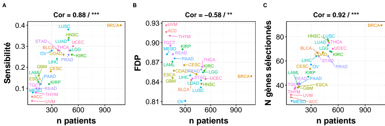
FIGURE 2.19 – Sensibilité (A), FDP (B), et nombre de gènes sélectionnés (C) en fonction du nombre de patients dans le jeu d'apprentissage sur les 26 cancers de TCGA étudiés et la pénalisation elastic net - données simulées.
