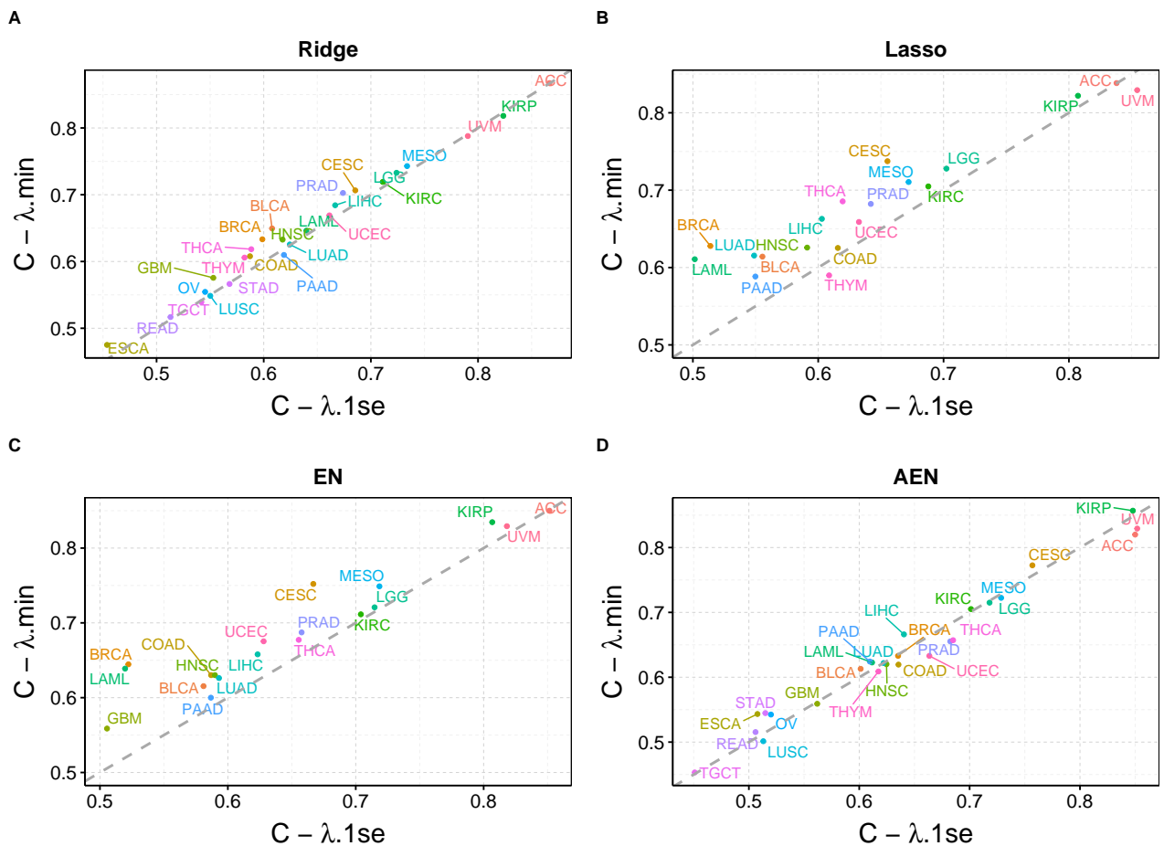
FIGURE 2.1 – C-index médians obtenus avec \lambda.min et \lambda.1se pour les quatre pénalisations et l'ensemble des 26 cancers de TCGA étudiés.
