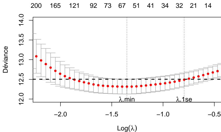
FIGURE 1.8 – Calcul du poids de la pénalité elastic net qui minimise la déviance globale. Les données d'expression d'ARN messagers de TCGA pour le cancer du rein à cellules claires (KIRC) sont utilisées.
