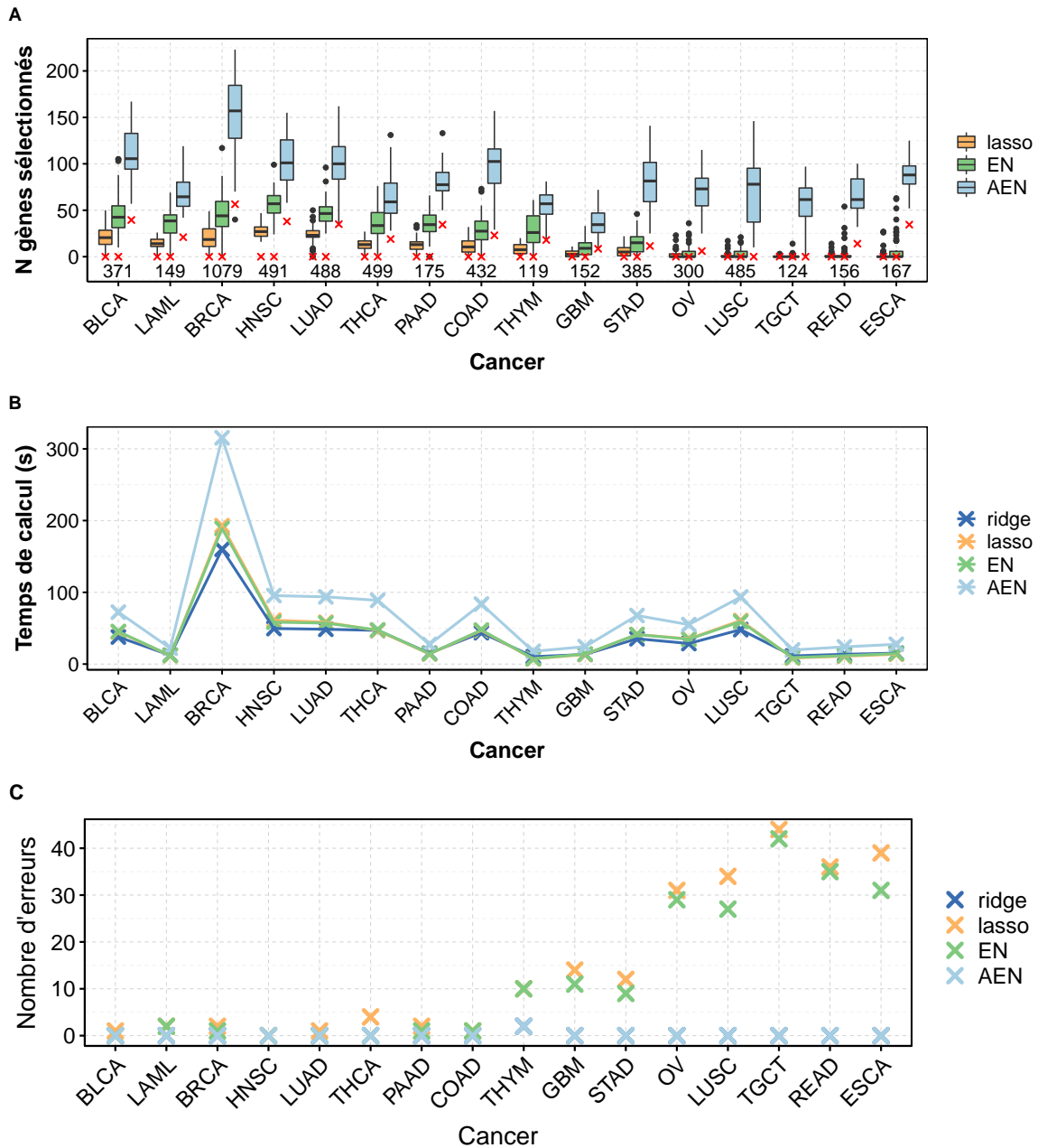
FIGURE A.4 – Nombre de gènes sélectionnés (A), temps de calcul médian (s) (B), et nombre d'erreurs dans le calcul du C-index avec \lambda_{\min} (C) des méthodes de pénalisation obtenus avec les données mRNA-seq.
