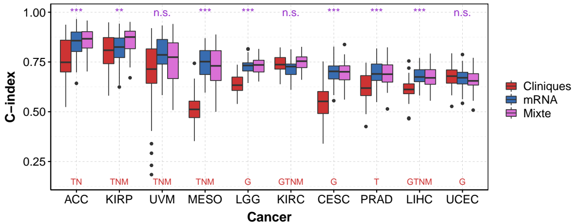
FIGURE 2.5 – C-index obtenus avec les données cliniques, mRNA-seq, et en mixant les deux types de données.
