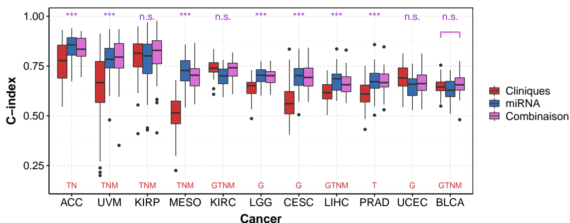
FIGURE 4.5 – C-index obtenus avec les données cliniques, miRNA-seq, et en combinant les deux types de données pour les 11 cancers étudiés.
