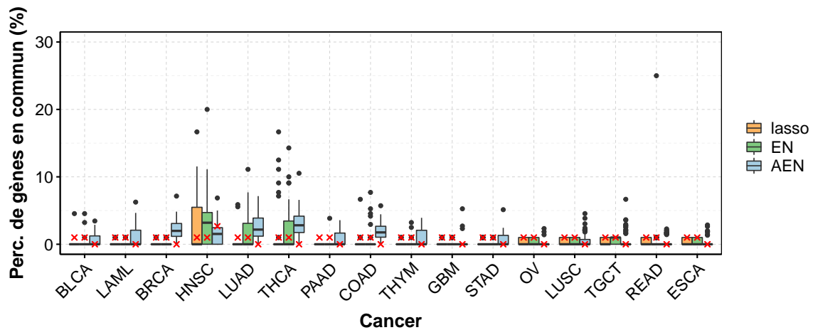
FIGURE A.9 – Stabilité des gènes sélectionnés.
