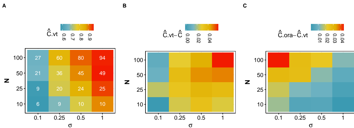
FIGURE 2.20 – C-index médians obtenus si la vérité terrain était connue (A), et différences médianes avec les C-index obtenus avec l'ensemble des gènes (B), et avec les C-index oracles (C) pour elastic net et LGG - données simulées.
