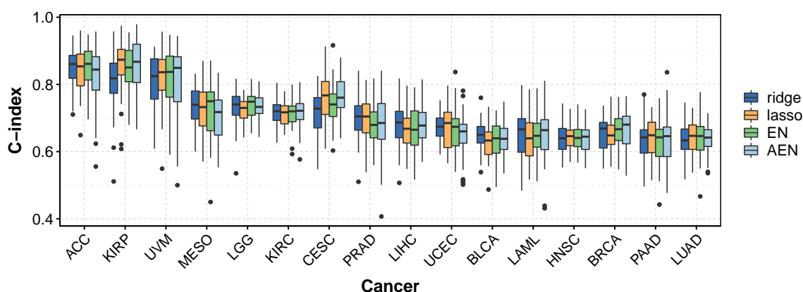
FIGURE 3.5 – C-index obtenus après pré-filtrage pour les quatre méthodes de pénalisation ( i.e. ridge, lasso, elastic net et adaptive elastic net) et 16 cancers de TCGA.
