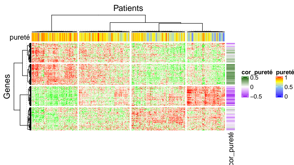
FIGURE 5.5 – Heatmap du niveau d'expression standardisé des gènes pour BLCA, et corrélation avec la pureté de la tumeur.
