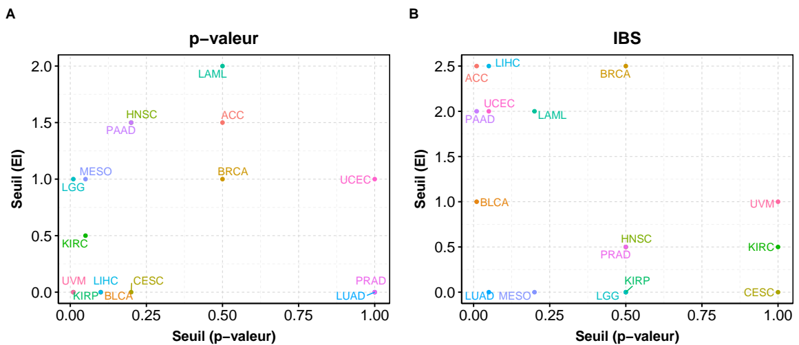
FIGURE A.11 – Seuils optimaux pour la pénalisation elastic net, l'ensemble des 26 cancers, et la p-valeur du modèle de Cox univarié (A) et l'IBS (B).
