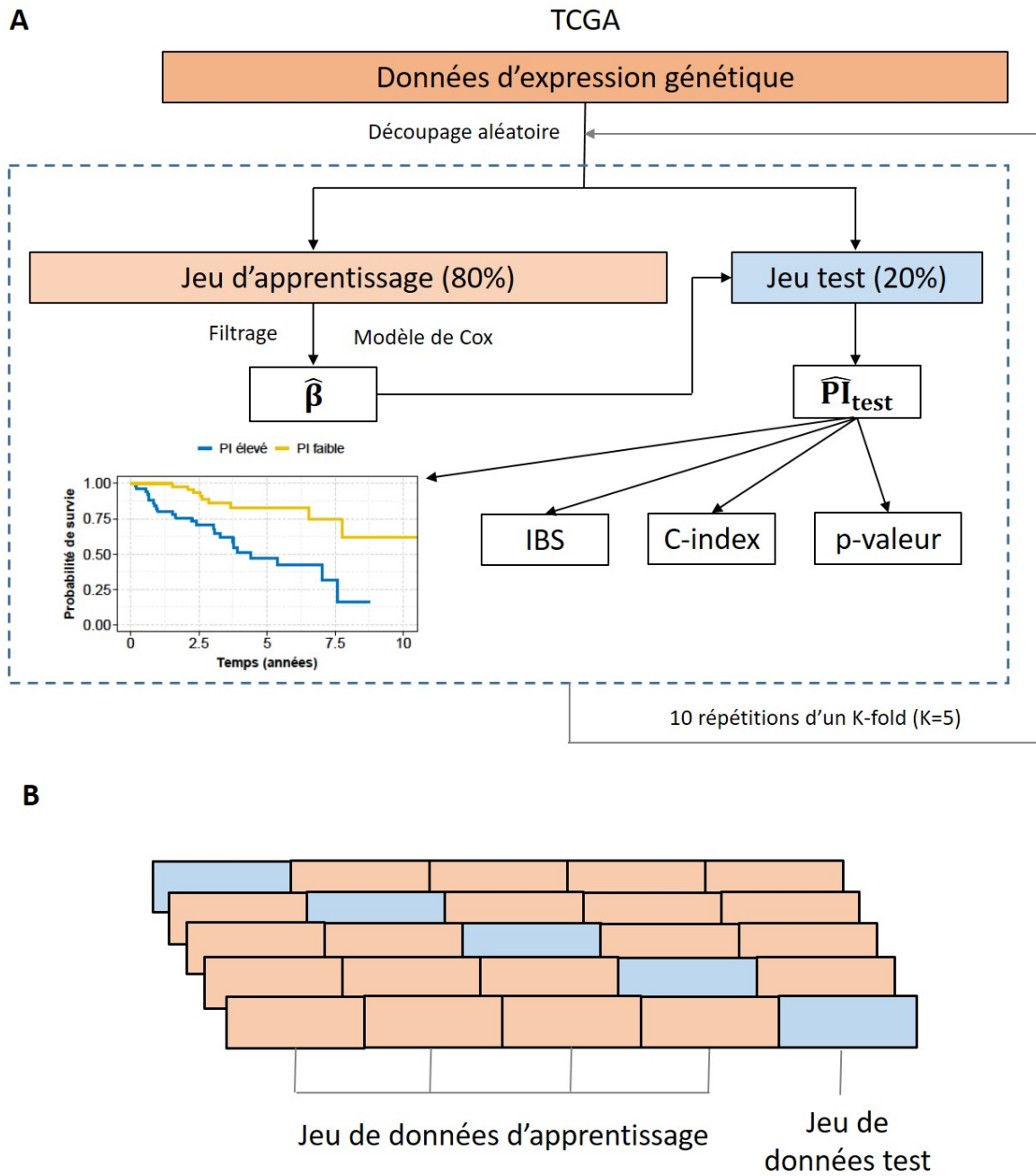
FIGURE 1.6 – Schéma récapitulatif de l'évaluation des modèles de prédiction.
