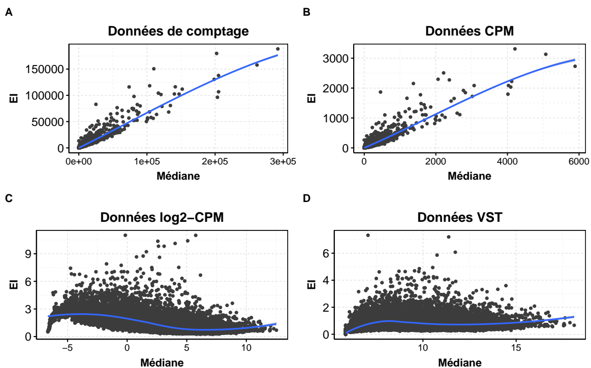
FIGURE 3.1 – Relation entre l'écart interquartile et la médiane dans les données de comptage RNA-seq (A), CPM (B), log2-CPM (C), et VST (D) pour LGG.
