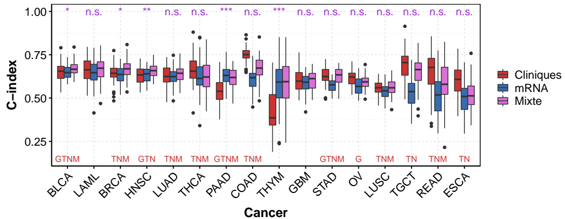
FIGURE A.5 – C-index obtenus avec les données cliniques, mRNA-seq, et en mixant les deux types de données.
