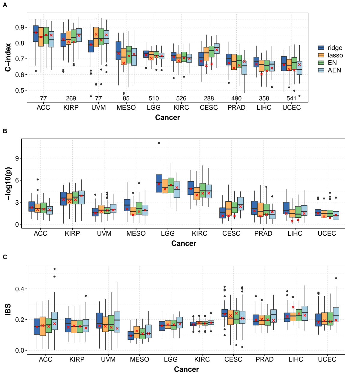
FIGURE 2.3 – C-index (A), p-valeurs du modèle de Cox univarié ( -\log_{10} ) (B), et IBS (C) obtenus avec les données mRNA-seq.
