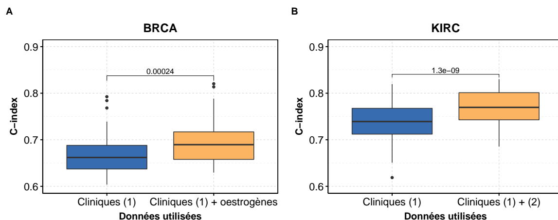
FIGURE 5.2 – C-index obtenus après l'ajout de nouvelles variables cliniques pour BRCA (A) et KIRC (B).
