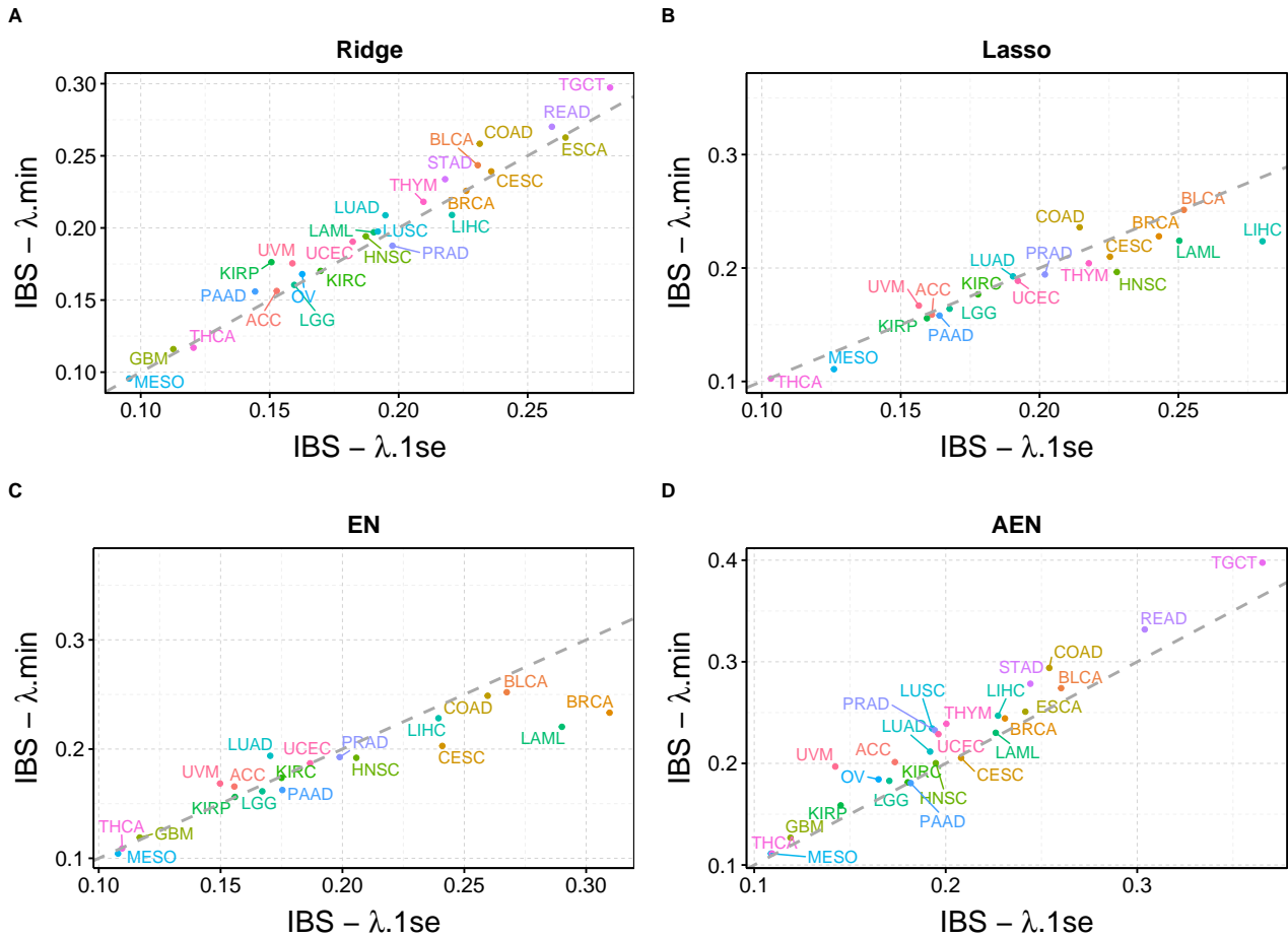
FIGURE A.2 – IBS obtenus avec \lambda.\min et \lambda.1se pour les quatre pénalisations et l'ensemble des 26 cancers de TCGA étudiés.
