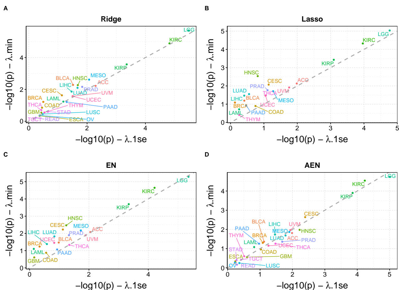
FIGURE A.1 – P-valeurs médianes du modèle de Cox univarié ( -\log_{10} ) obtenues avec \lambda_{\min} et \lambda_{1se} pour les quatre pénalisations et l'ensemble des 26 cancers de TCGA étudiés.
