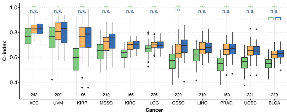
FIGURE 4.9 – Evaluation des deux hypothèses pour expliquer la diminution des capacités de prédiction induite par la dégradation des données miRNA-seq des 11 cancers étudiés.
