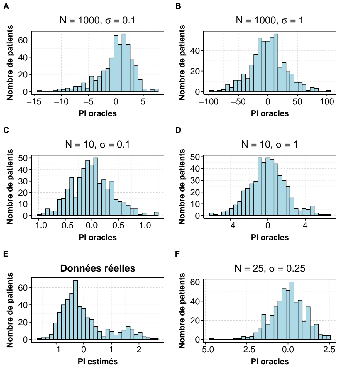
FIGURE 2.7 – Histogrammes des indices pronostiques oracles obtenus avec différents paramètres de simulation et sur données réelles pour LGG.
