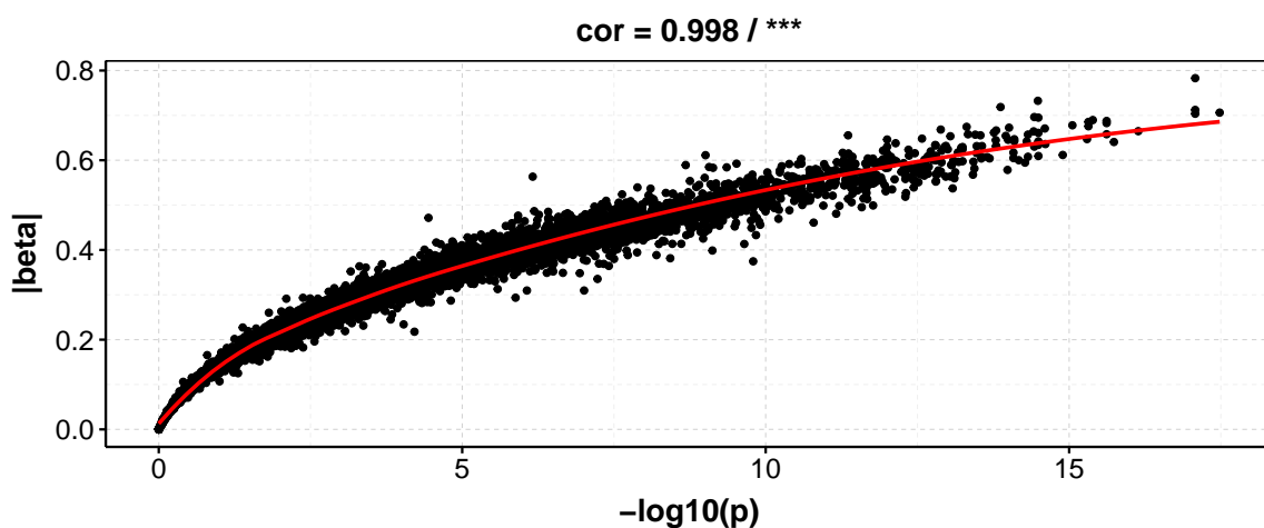
FIGURE 3.6 – Valeurs absolues des coefficients \beta en fonction des p-valeurs en échelle -\log_{10} d'un test du rapport de vraisemblance corrigées par la méthode de Benjamini-Hochberg calculés à partir d'un modèle de Cox univarié pour LGG.
