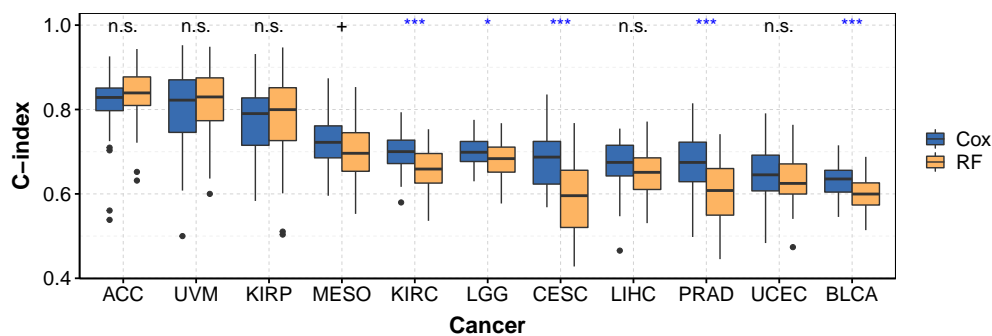
FIGURE 5.6 – C-index obtenus avec le modèle de Cox pénalisé (ridge, bleu) et un algorithme de forêts aléatoires (jaune) sur les données miRNA-seq.
