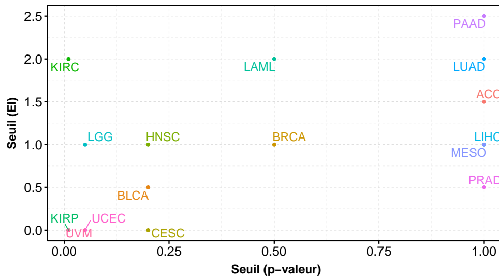
FIGURE 3.3 – Seuils optimaux pour la pénalisation elastic net, le C-index, et l'ensemble des 16 cancers.
