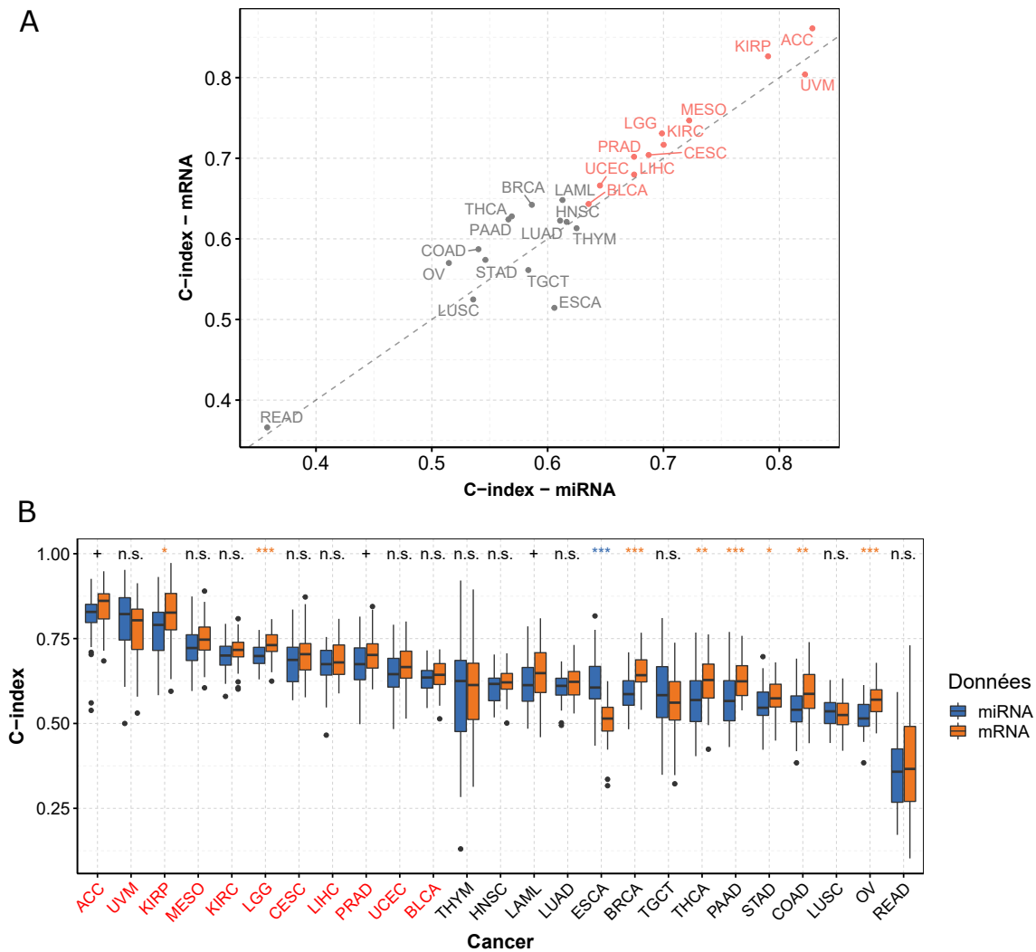
FIGURE 4.4 – C-index obtenus avec les données RNA-seq pour les ARNm et les miARN pour 25 cancers de TCGA
