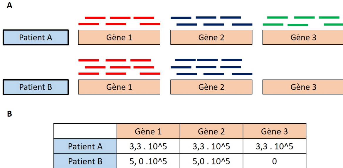
FIGURE 1.3 – Exemple de biais induit par la normalisation CPM
