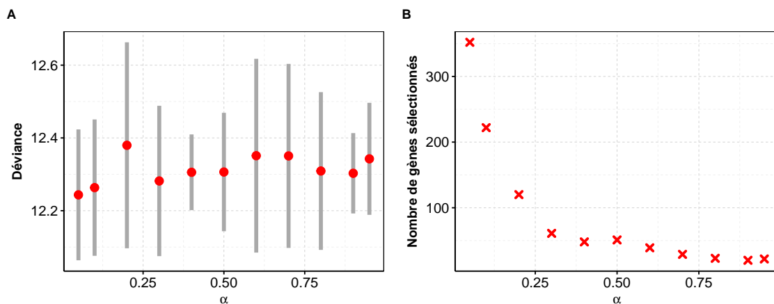
FIGURE 1.9 – Déviance globale (A) et nombre de gènes sélectionnés (B) pour différentes valeurs de \alpha dans la pénalisation elastic net pour les données mRNA-seq de KIRC.
