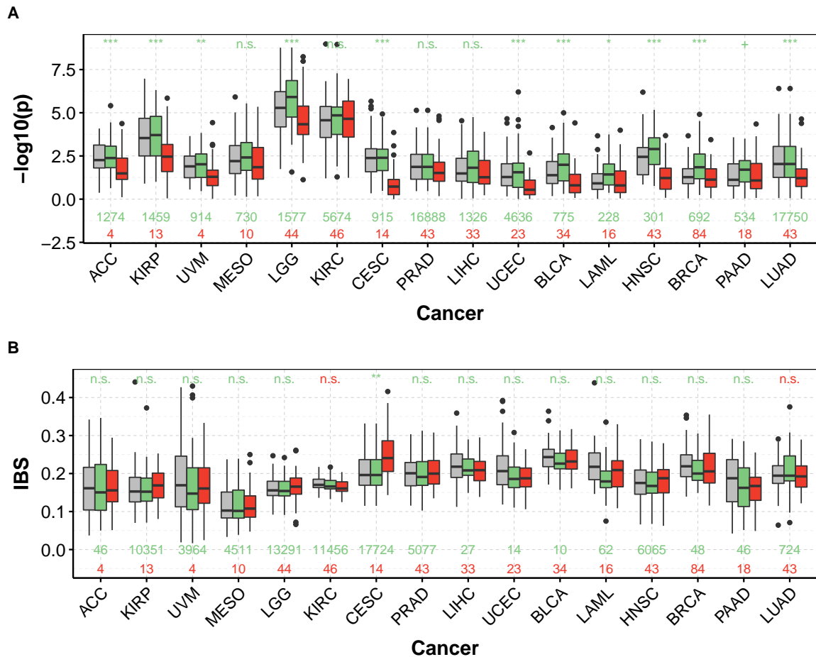
FIGURE A.12 – P-valeurs du modèle de Cox univarié ( -\log_{10} ) (A) et IBS (B) obtenus sans pré-filtrage (gris), avec le pré-filtrage bi-dimensionnel et la pénalisation elastic net (vert), et avec l'algorithme ISIS (rouge) pour 16 cancers de TCGA.
