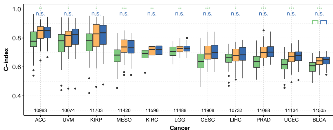
FIGURE A.15 – Cause de la diminution des capacités de prédiction induite par la dégradation des données mRNA-seq des 11 cancers étudiés.
