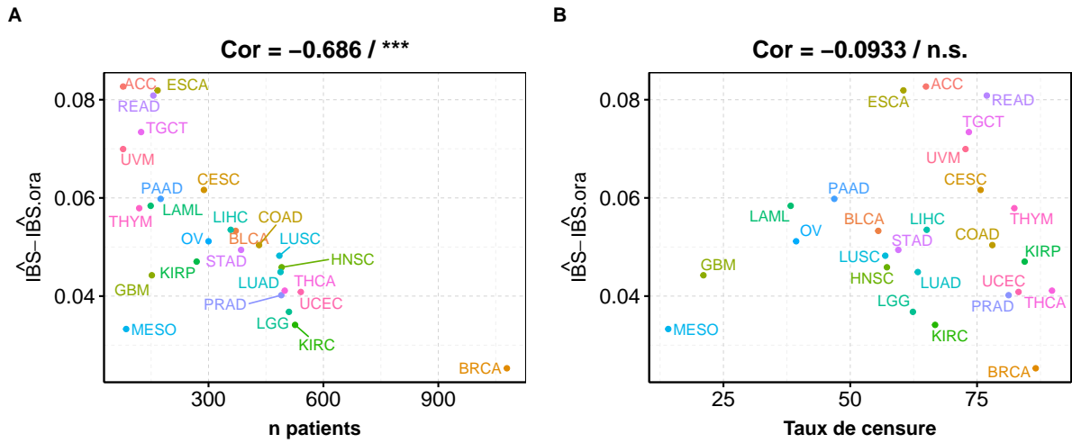
FIGURE A.8 – Différences médianes entre les IBS estimés et oracles en fonction du nombre de patients (A) et du taux de censure (B) pour l'ensemble des 26 cancers étudiés.
