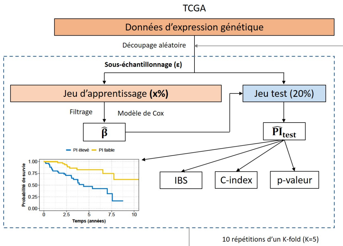
FIGURE 4.6 – Procédure d'évaluation de l'impact de la dégradation des données de comptage RNA-seq et du nombre de patients sur la prédiction.
