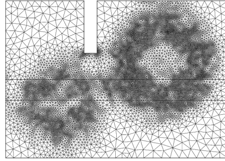
FIGURE 8.6 – Premier niveau de raffinement (23238 triangles)
