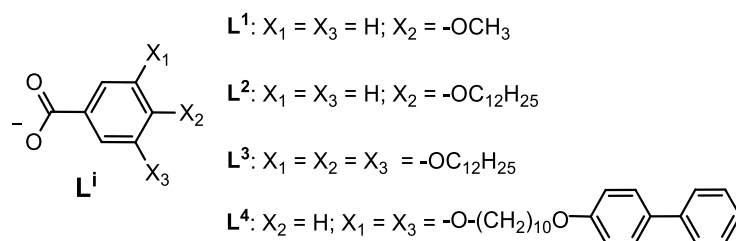
Schéma R-1. Structure chimique des ligands L^{1-4} utilisés pour la fonctionnalisation des sites équatoriaux du complexe Mn_{12} .
