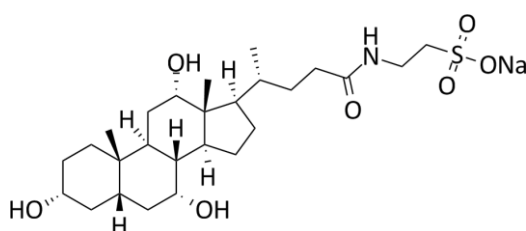
Figure 53 : Structure du taurocholate de sodium.
