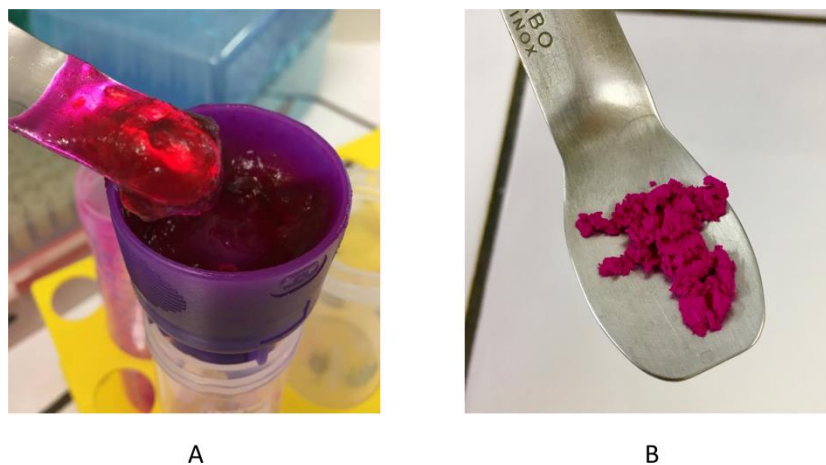
Figure 76 : PLL-rhodamine 52 kD obtenue. (A) après ajout de 10 éq. de DIEA et 0,1 éq. de RBITC pour 1 éq. de PLL (B) après ajout de 2,5 éq. de DIEA et 0,05 éq. de RBITC pour 1 éq. de PLL.
