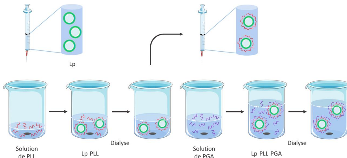
Figure 31 : Procédure de formulation des liposomes recouverts de 2 couches de polyelectrolytes ou layersomes.
