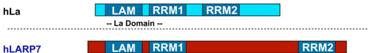
Figure 13 : domaines structuraux des protéines La et Lar7. LAM : La Motif ; RRM : RNA Recognition Motif (Bayfield et al., 2010).
