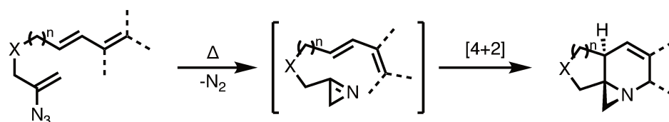
Figure 1.25 Réaction d'aza-IMDA
