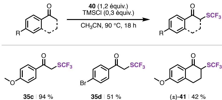
Figure 2.5 Synthèses de cétones de départ avec le réactif de Billard de seconde génération
