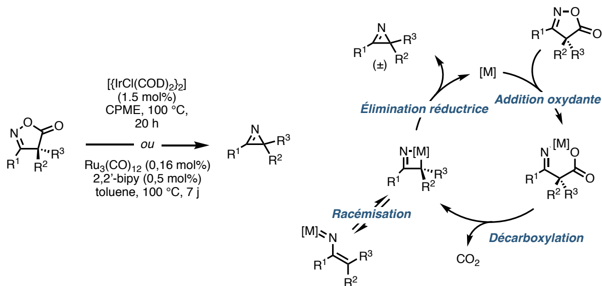
Figure 1.6 Synthèse de 2 H -azirines à partir d'isoxazol-5(4 H )-ones
