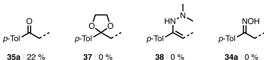
Figure 2.2 Premières tentatives de synthèse des cétones de départ (phen = phénantroline)
