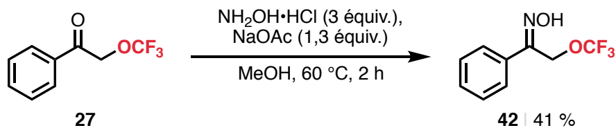
Figure 2.7 Synthèse de l'oxime 42
