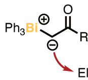
Figure 2.4 Principales applications des composés de Bi(V)
