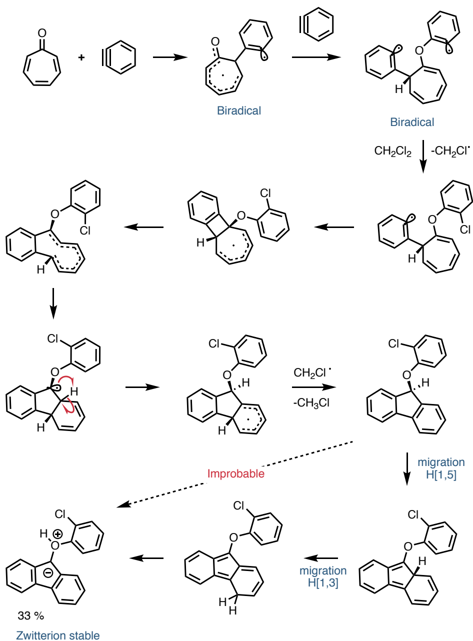
Figure 1.13 Réaction entre la troponone et le benzyne
