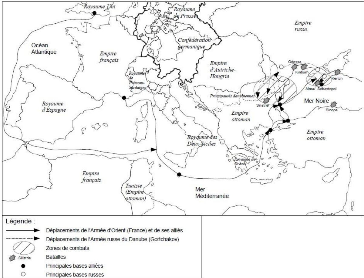
Carte n°1 : La guerre de Crimée en mer Méditerranée et en mer Noire
