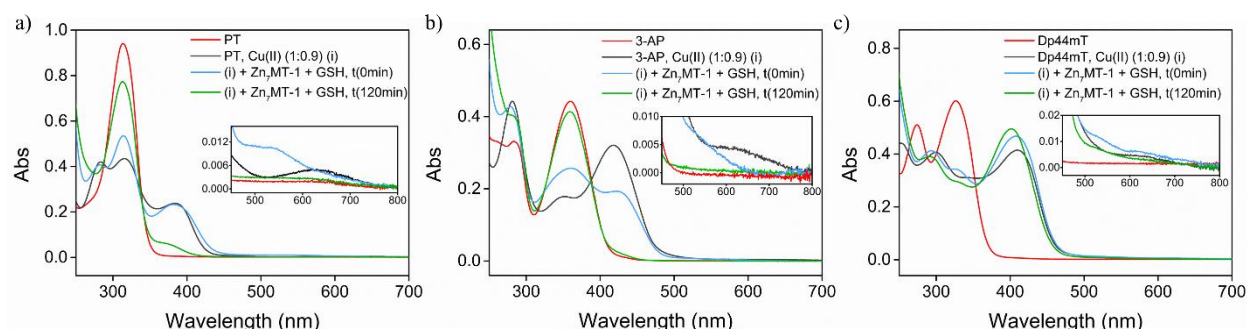
Image 5 - Spectres UV-Vis permettant le suivi de la réaction de a) Cu(II)-PT, b) Cu(II)-3-AP et c) Cu(II)-Dp44mT avec GSH/Zn(II) 7 MT-1 à 0 et 120 min après addition de GSH et de Zn(II) 7 MT-1 aux complexes Cu(II)-TSC préformés. Conditions expérimentales: L 30 \mu M, Cu(II) 27 \mu M (1:1:1), GSH 3 mM, Zn(II) 7 MT-1 6 \mu M, tampon HEPES 100 mM, pH 7.4.
