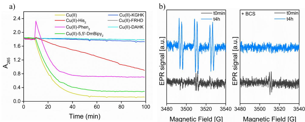
Image 4 - a) Évolution dans le temps de l'absorption de AscH• à \lambda_{\max} = 265 nm, après addition au temps t = 10 min de Cu(II) libre ou de complexes de Cu(II). Les concentrations initiales en Cu(II), peptide/ligands, AscH• et H 2 O 2 étaient respectivement de 10 \mu M, 12 \mu M/24 \mu M, 100 \mu M et 100 \mu M dans du PB 50 mM, pH 7.4. b) Mesure indirecte de la production de HO• par RPE avec piégeage de spin, en utilisant POBN comme premier piègeur de spin, en présence (panneau de droite) et en absence (panneau de gauche) de BCS. Conditions expérimentales: KGHK 120 \mu M, Cu(II) 100 \mu M (1.2:1), AscH• 1 mM, H 2 O 2 1 mM, PB 100 mM, pH 7.4, POBN 50 mM, ETOH 5%, BCS 300 \mu M.
