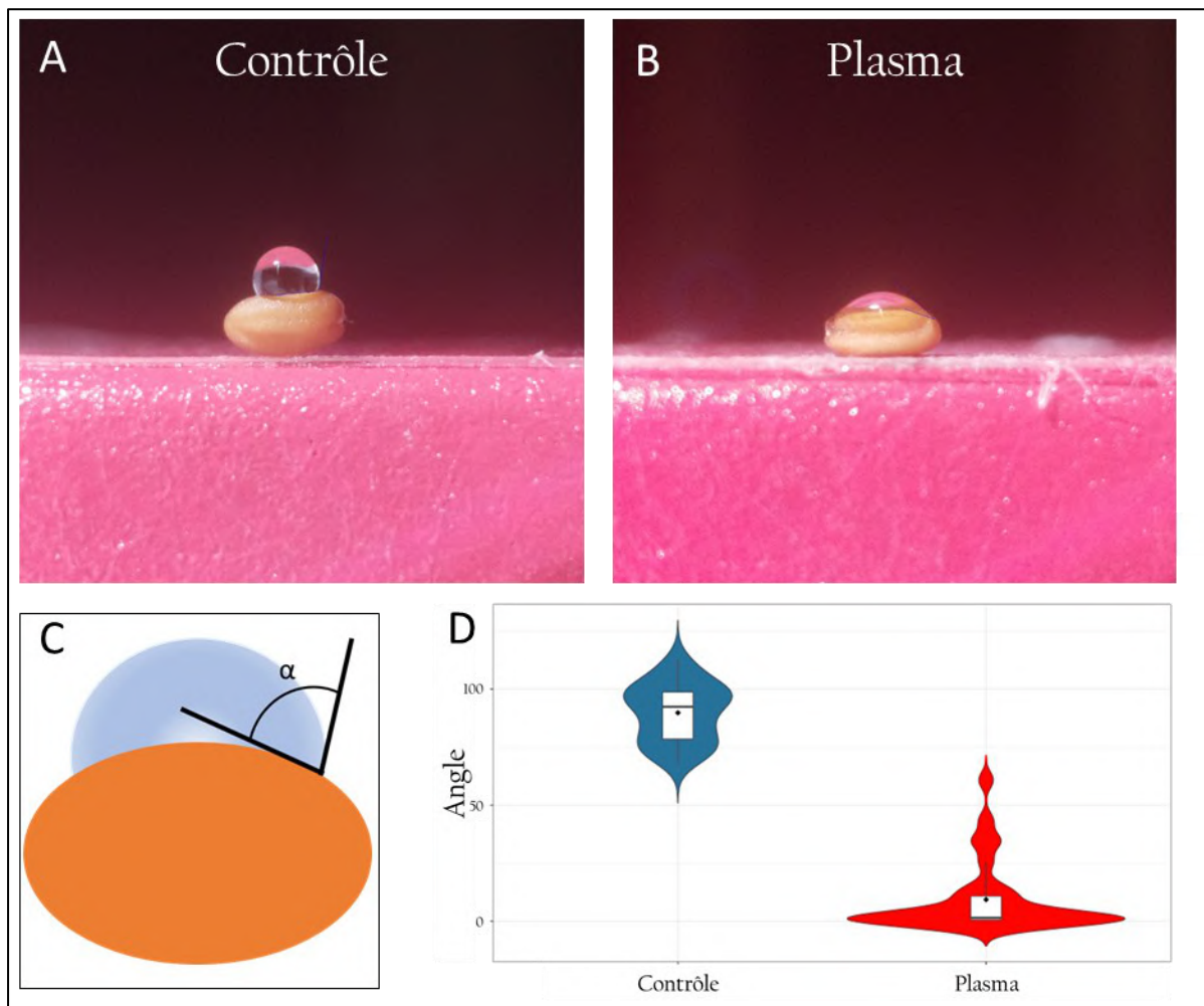
Figure III-13 : Le traitement au plasma diminue l'angle de contact des graines de Camelina sativa . Photos des graines de C. sativa après dépôt de la goutte de 0.3 \mu L. Graine contrôle (A), ou traitée grâce à la FE-DBD pendant 15 min (B). Schéma du calcul de l'angle de contact \alpha (C). Violin plot des mesures d'angles de contact sur 30 graines par traitement (D).
