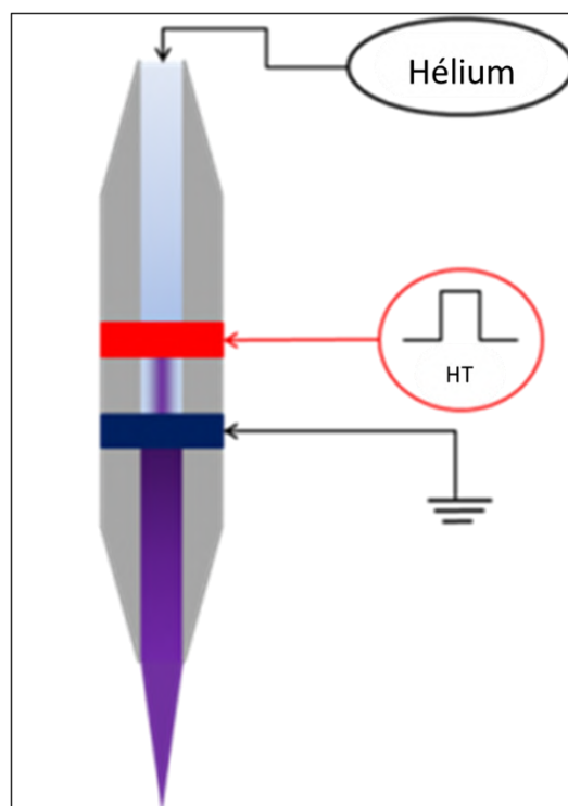
Figure II-2: Schéma du dispositif de jet de plasma d'hélium. Adapté de Bafail et al, 2018 [90]. Le gaz injecté dans le dispositif, ici l'hélium, est ionisé grâce aux électrodes et passe de l'état gazeux (en bleu) à l'état plasma (en violet).
