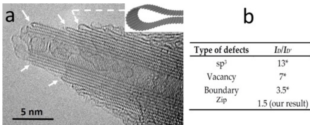
Figure 7 : (a) Image MET en résolution atomique de l'apex nanométrique d'un cône de carbone. Plusieurs exemples de paires de graphènes refermées l'une sur l'autre ("zippées") sont fléchés. La flèche pointillée désigne un défaut différent (en "boucle"), dont un modèle est donné en encart (Crédit image : R. Wang, CEMES). (b) Rapports des intensités des bandes Raman D et D' pour différents types de défauts, dont le défaut "zip" identifié dans notre travail. Les autres valeurs proviennent de [Eckmann et al., Nanolett. 12 (2012) 3925].
