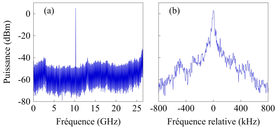
Figure I.16 – Spectres électriques du laser DFB-10G enregistrés à T = 19 \text{ }^\circ\text{C} et à P_{\text{pompe}} = 136 \text{ mW} . (a) Span : 26,5 GHz, RBW : 5 MHz. (b) Span : 1,6 MHz, RBW : 20 kHz.
