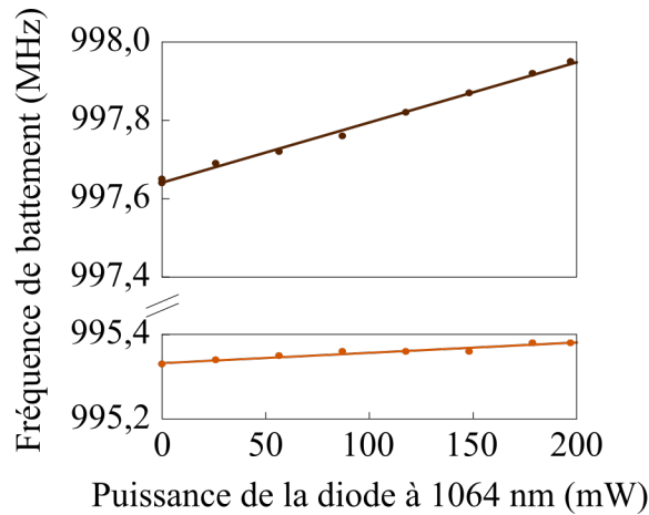
Figure I.26 – Variation de la fréquence de battement du laser DFB-1G-bis en fonction de la puissance de sortie de la diode à 1064 nm pour deux orientations de la polarisation de cette dernière. Pentés de 1,5 kHz/mW (courbe marron) et 0,2 kHz/mW (courbe orange).
