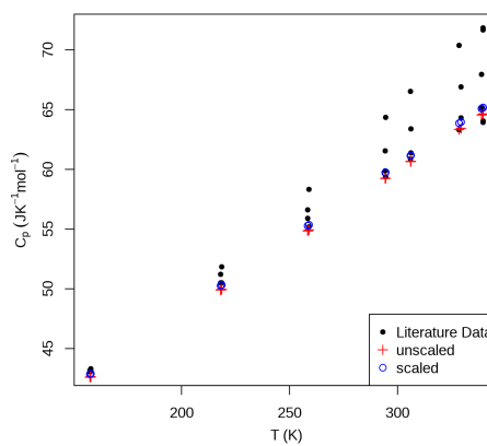
(d) propyne
