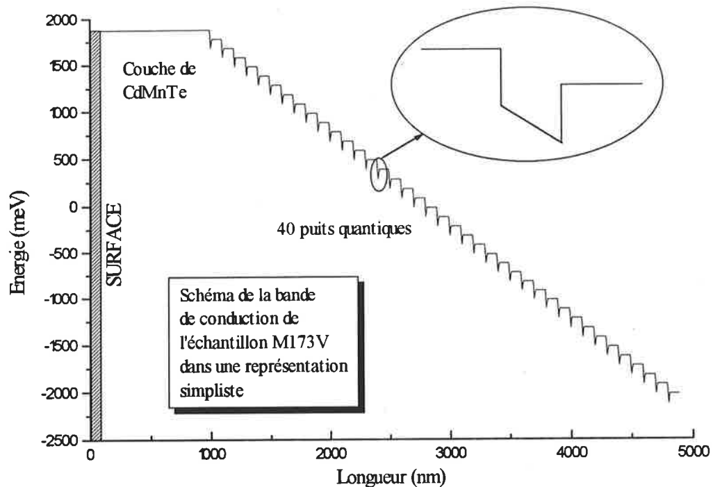
Figure IV-7 représentation schématique de la bande de conduction de l'échantillon M173V
