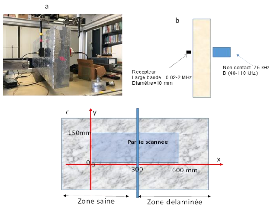
Figure III-14 : a) Dalle pendant le test de transmission sans contact b) explication symbolique de l'expériment c) la zone scannée
