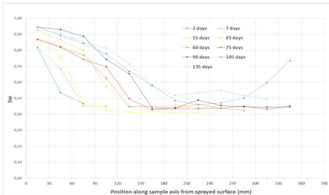
Figure IV-14 : Progression de la saturation dans des cylindres du même béton qui a servi pour la construction du mur, soumis à pulvérisation d'eau (comme pour le mur)
