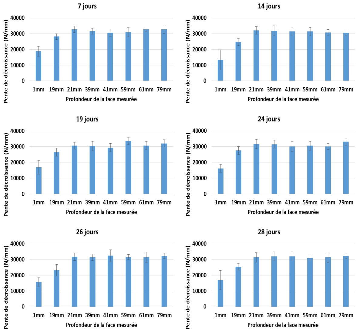
Figure A.II.3.2 : Évolution de la pente [Force/déplacement] sur essai de microindentation en fonction de la profondeur par rapport à la surface exposée à la solution lixiviante en fonction du temps d'exposition au nitrate d'ammonium pour chaque tranche issue des carottages
