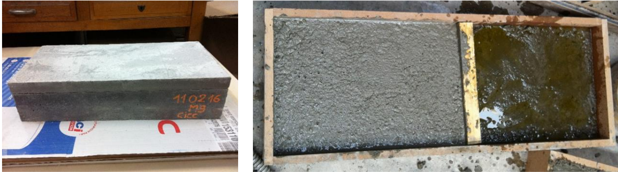
Figure III-3 : [gauche] Cinquième dalle de la série 1, composée d'une dalle de 3 cm d'épaisseur et une dalle de 9cm d'épaisseur, superposée ; [Droite] dalle de la série 2 : mise en place de l'interface huilée
