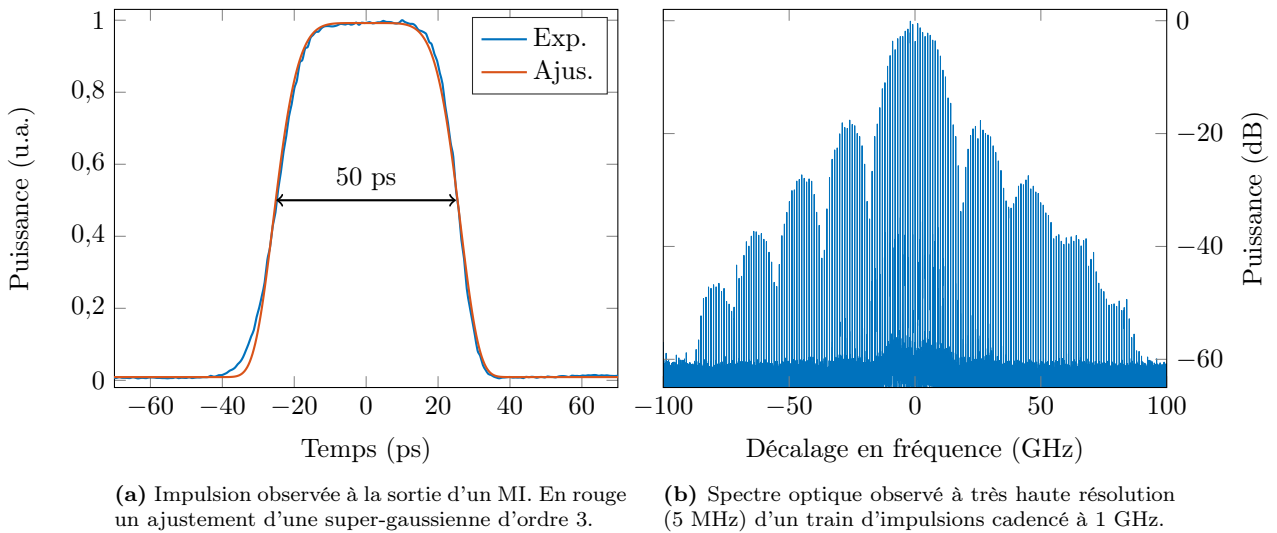
FIGURE 1.17 – Impulsion temporelle et spectre optique observables à la sortie du montage présenté à la Figure 1.16. Une impulsion super-gaussienne d'ordre 3 étant proche d'une impulsion porte, son spectre est déjà très proche d'un sinus cardinal.
