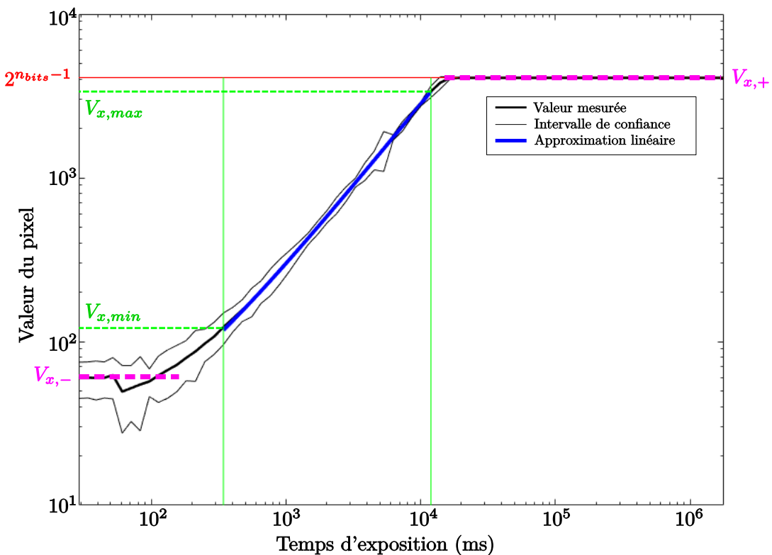
FIGURE 5.37 – Analyse d'une courbe de calibration r_x . On cherche à définir les limites de sur- et sous-exposition ( V_{x,min} et V_{x,max} ) permettant d'établir un domaine de bonne bijectivité de r_x . Pour cela, on estime les niveaux de saturation bas V_{x,-} et haut V_{x,+} , puis on réduit l'intervalle jusqu'à ce qu'une approximation linéaire (bleu) soit correcte, avec moins de 10% d'erreur.
