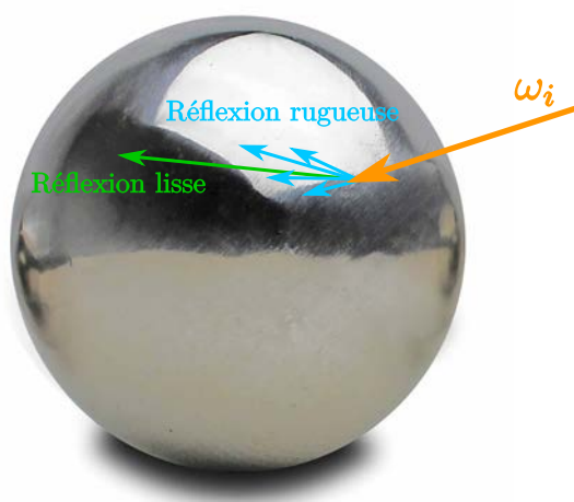
FIGURE 3.16 – Rayures et non-uniformités du matériau. La diffusion de la lumière dépend de l'endroit où celle-ci impacte l'objet, ce qui va à l'encontre des hypothèses de mesure.
