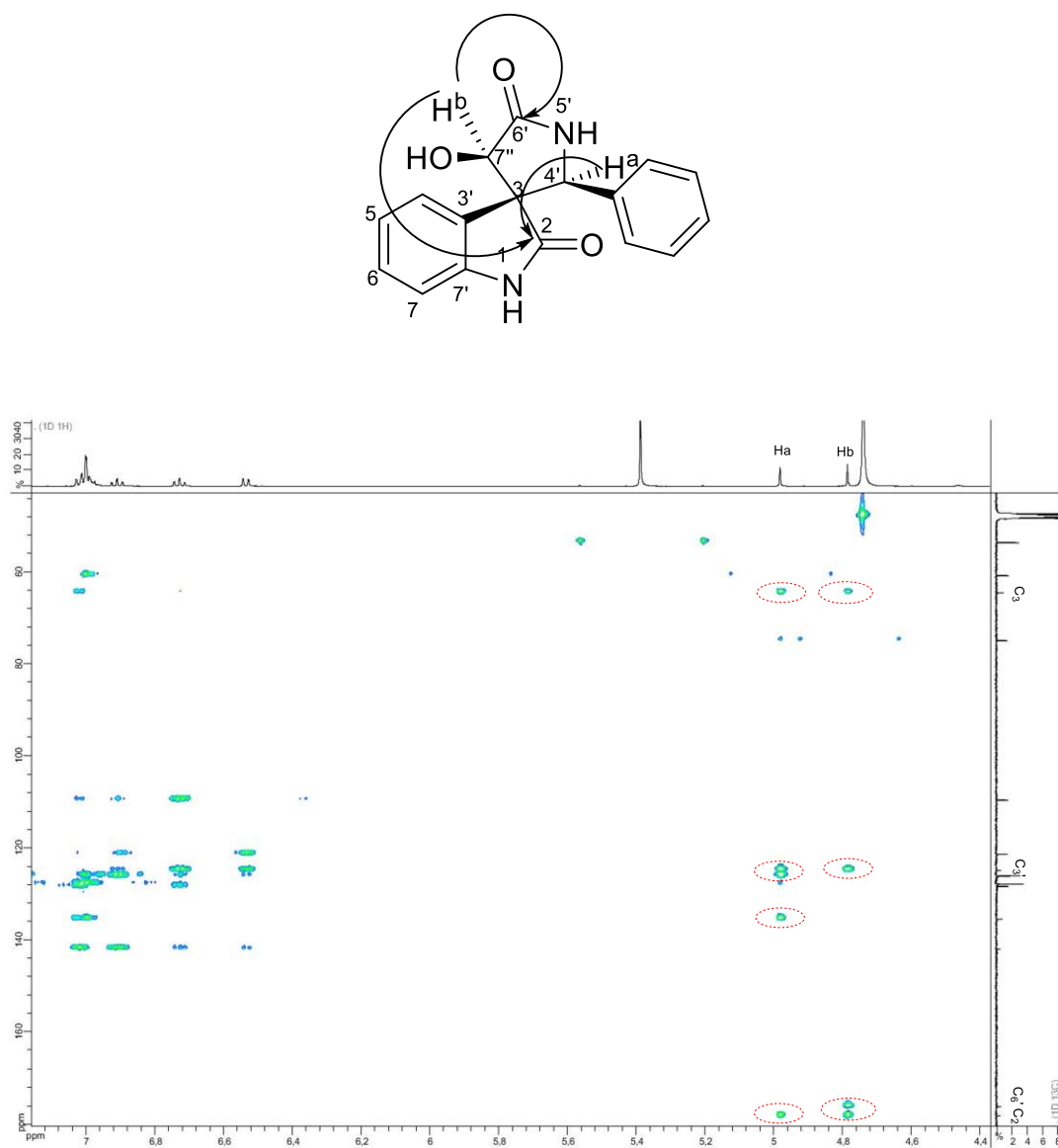
Figure 23. Analyse HMBC de composé 120 montrant des corrélations entre H^a (protons benzylique) et C_3 (carbone spiro), H^a et C_2 (carbonyle de l'oxindole), H^b (proton \alpha de l'hydroxyle) et C_2 , H^b et C_6 (carbonyle de l'hydroxy lactame), et entre H^a , H^b et C_3 .
