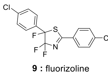
Figure 5. Structure de la fluorizoline ( 9 ). 20
