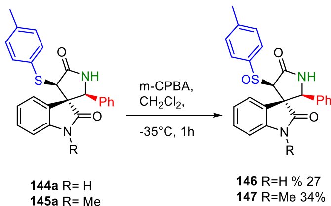
Schéma 29. Oxydation des composés 144a et 145a par du m -CPBA.
