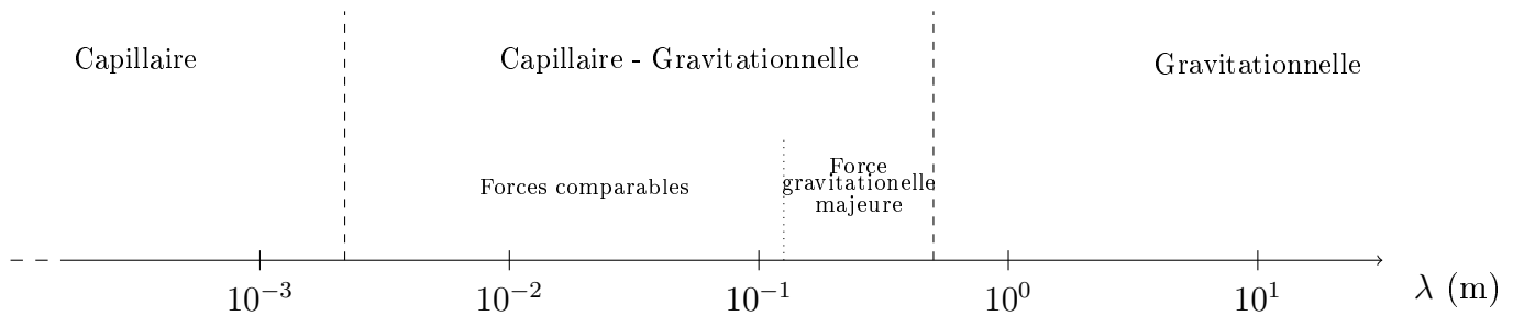
Figure 2.4. – Type de vague en fonction de la longueur d'onde \lambda
