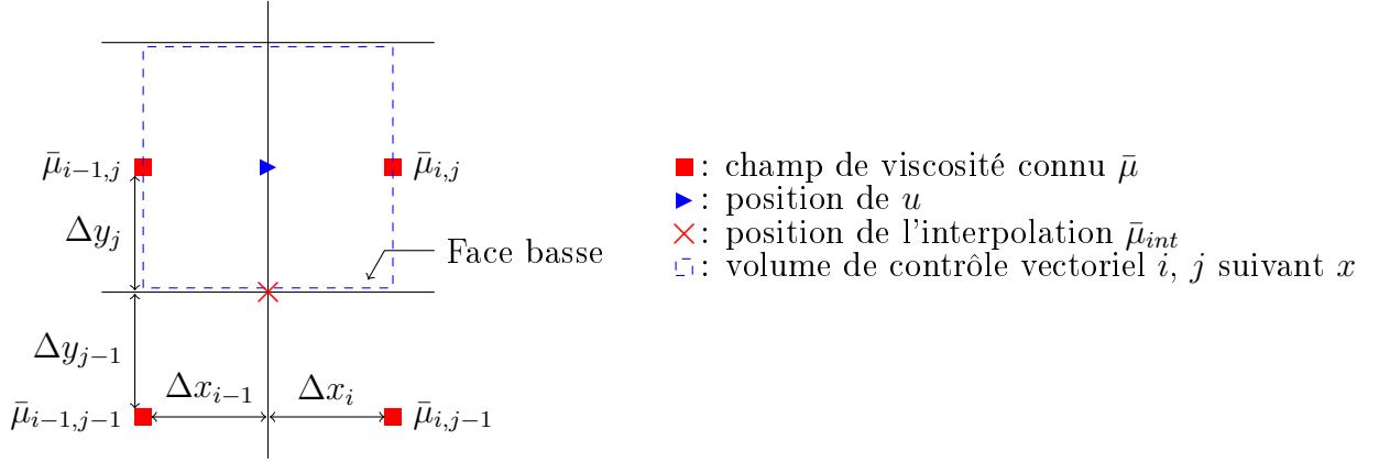
Figure 3.9. – Schéma de l'interpolation harmonique de la viscosité moyennée \bar{\mu} sur la face basse du volume de contrôle vectoriel suivant x .
