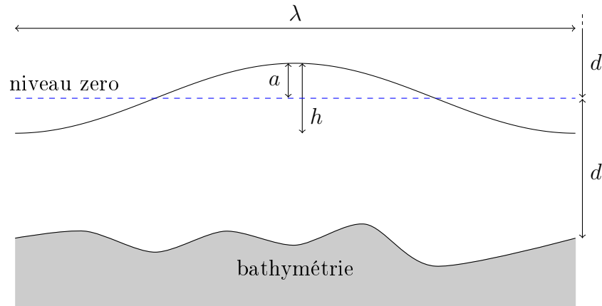
Figure 2.1. – Définition des grandeurs liées à une onde sinusoidale.
