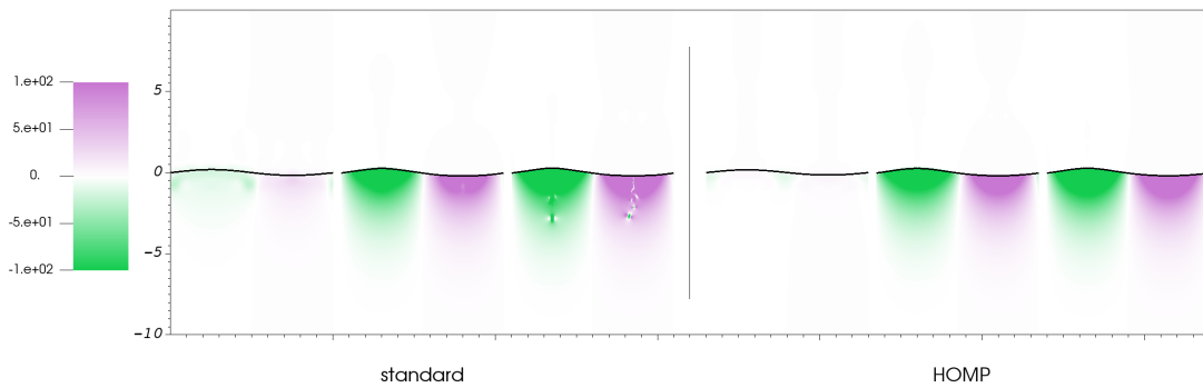
(c) WENO 5,3
