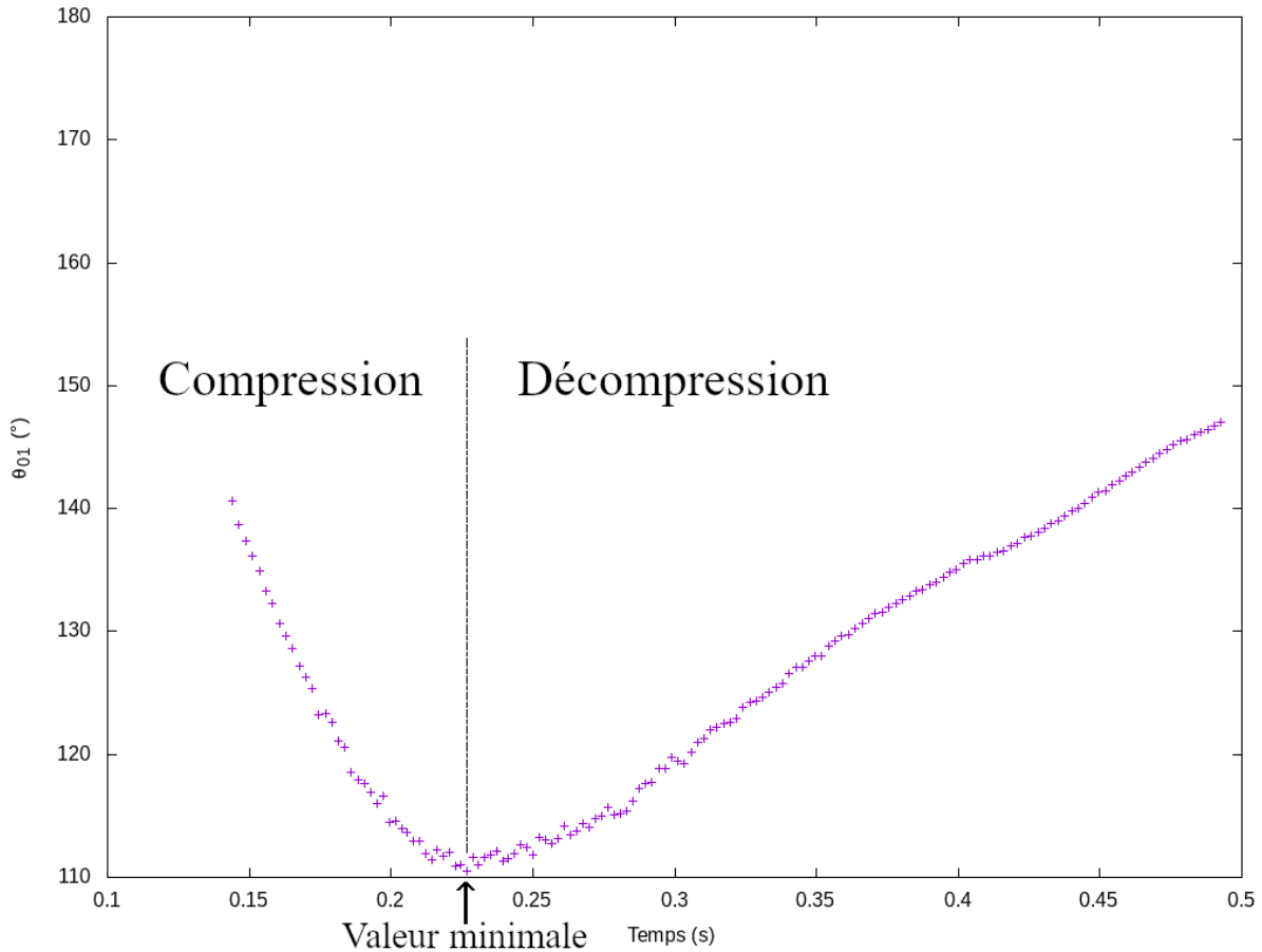
Figure 5.11. –  volution de \theta_{01} ( ) au cours du temps (s) pour la simulation correspondant aux conditions initiales : \frac{d}{\lambda} = 0.1 , \lambda = 0.05 m et \epsilon = 0.15 .
