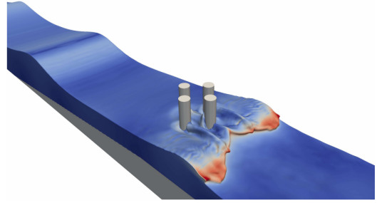
(b) Simulation numérique du déferlement d'une vague sur un groupe de quatre cylindres. L'image provient de l'article de M. A. Chella et al [43].
