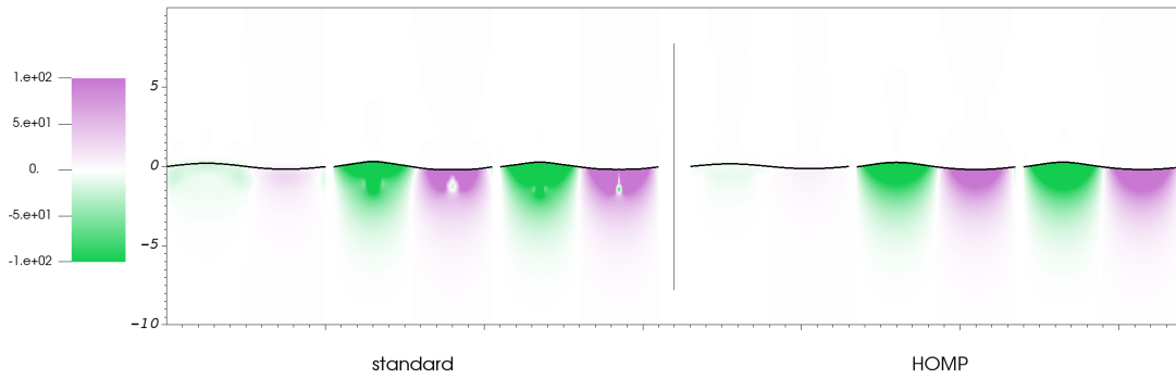
(b) WENO 3,2
