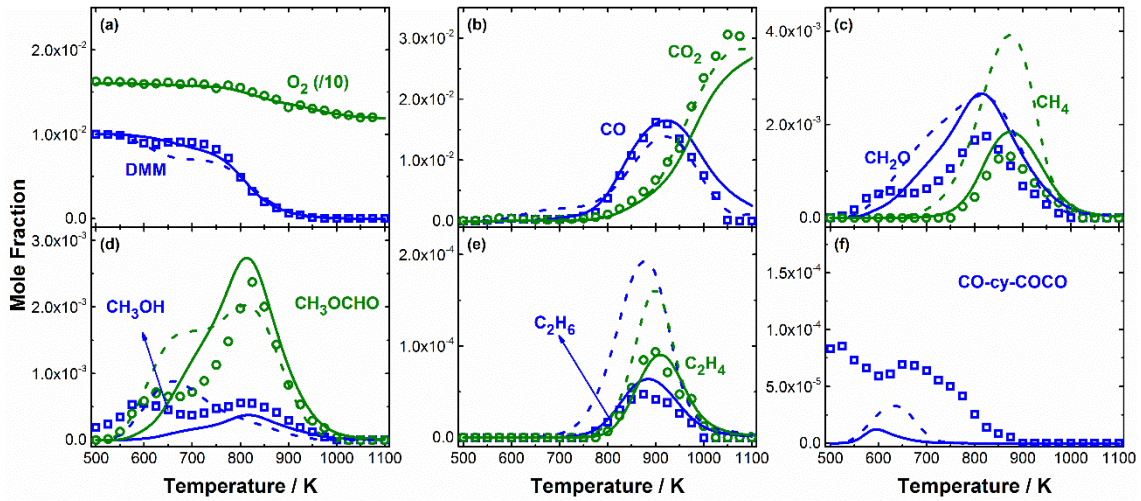
Figure VI. 4 : Comparaison des simulations obtenues avec notre modèle et celui de Vermeire et al. dans les conditions de l'étude de Vermeire et al. [132] en JSR ( \phi = 0.25 , P = 1.07 bar, \tau = 2.83 s); Symboles : mesures, lignes continues : notre modèle, lignes discontinues : modèle de Vermeire et al..
