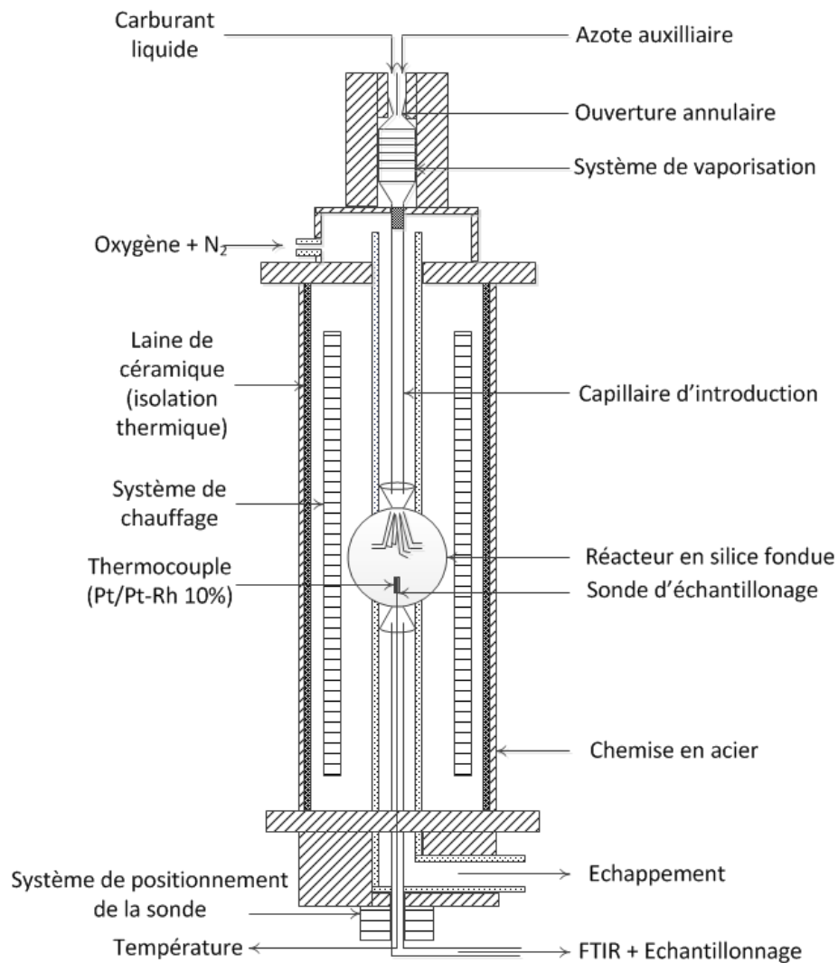
Figure III. 2 : Schéma du réacteur auto-agité d'Orléans.
