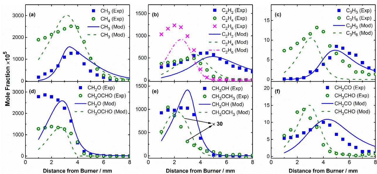
Figure VI. 14 : Comparaison des résultats expérimentaux (symboles) [211] et calculés (lignes) pour les produits intermédiaires mesurés dans une flamme laminaire de prémélange DMM/O 2 /Ar à basse pression.
