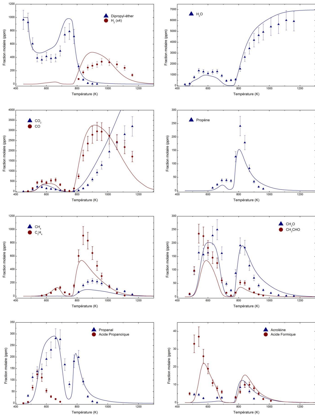
Figure V. 11 : Résultats obtenus pour l'oxydation de l'éther dipropylique à 10 atm et \tau = 0,7s pour 1000ppm de DPE initial à \phi = 0,5 .
