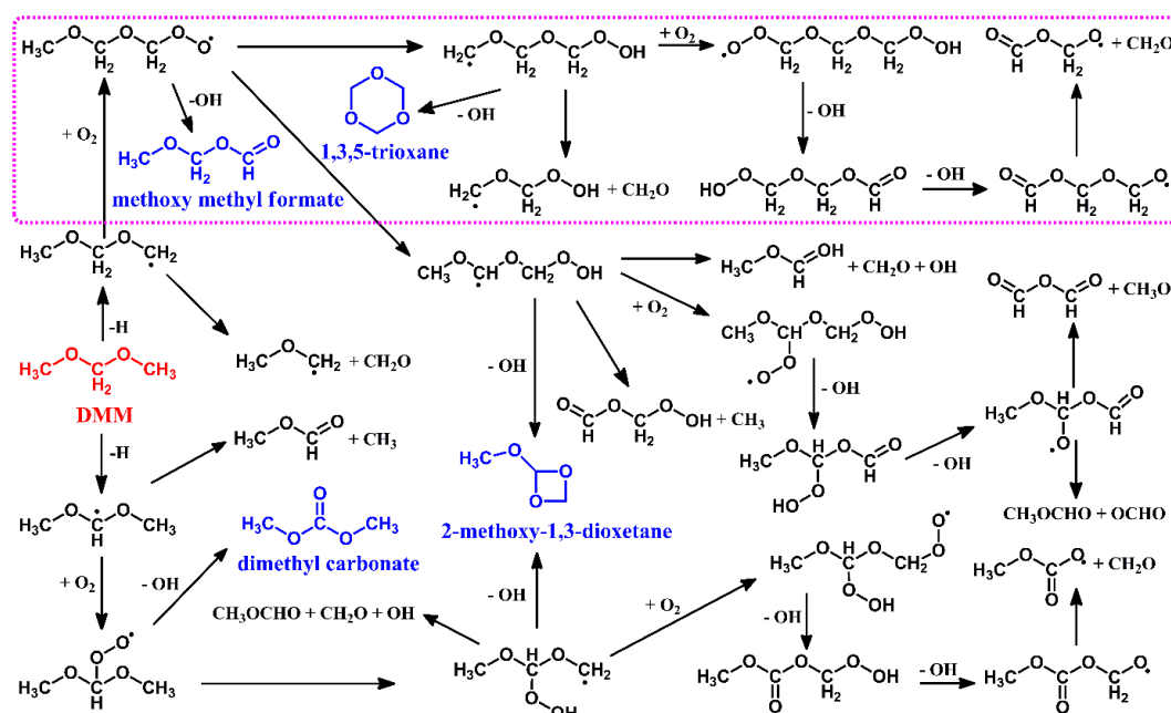
Figure VI. 1 : Schéma d'oxydation du DMM. Les espèces en bleu sont les isomères possibles correspondant à m/z 90.03.
