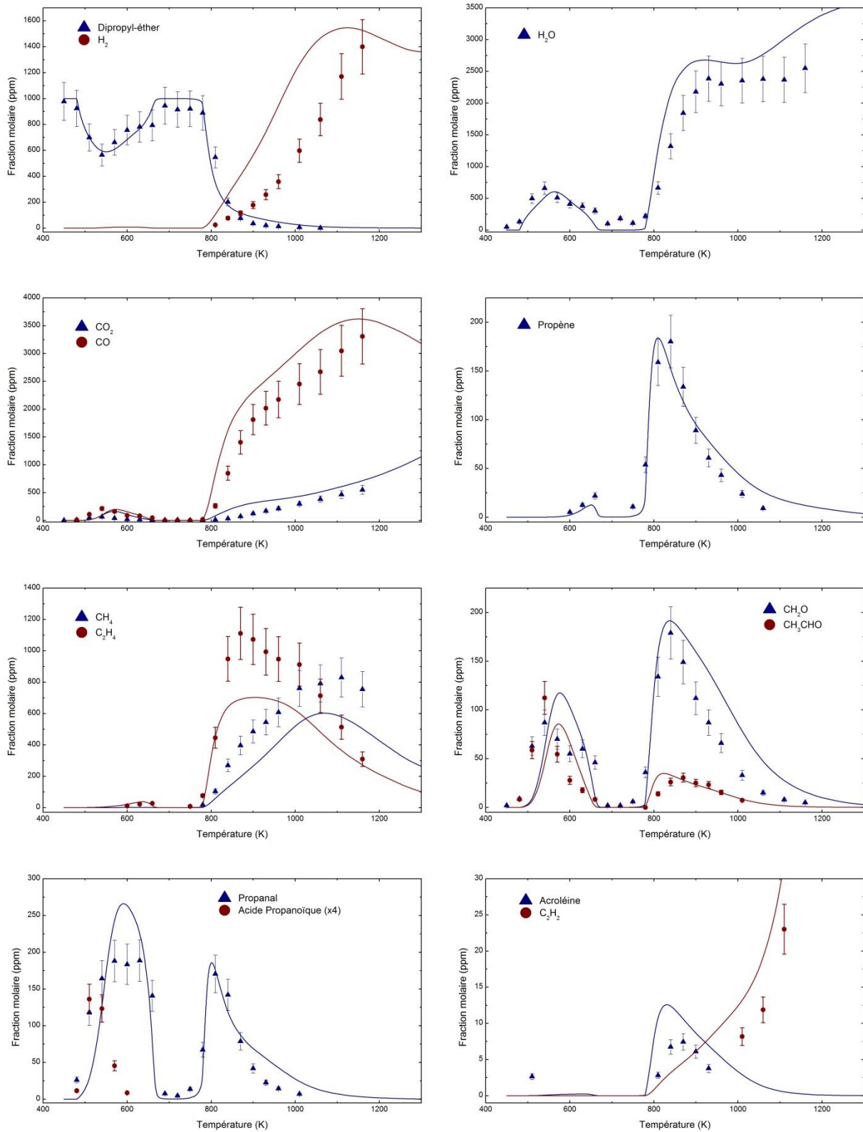
Figure V. 13 : Résultats obtenus pour l'oxydation de l'éther dipropylique à 10 atm et \tau = 0,7s pour 1000ppm de DPE initial à \phi = 2 .
