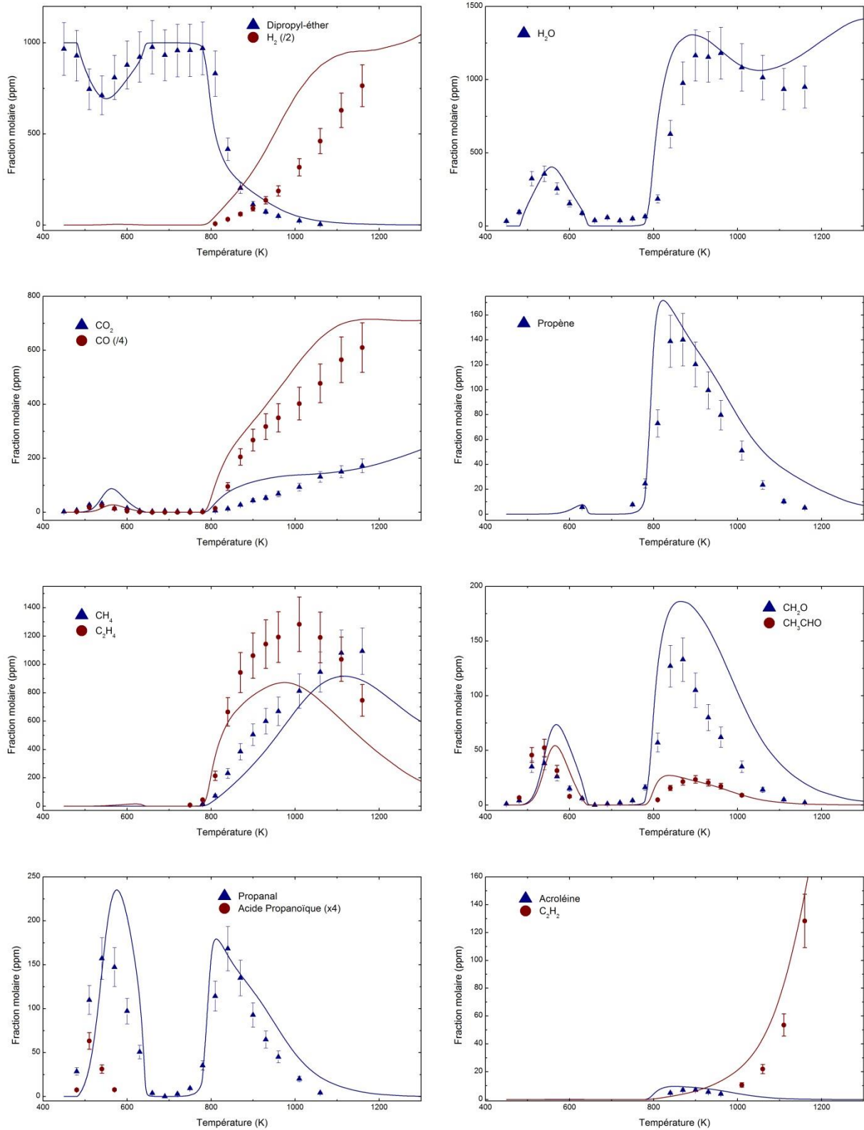
Figure V. 14 : Résultats obtenus pour l'oxydation de l'éther dipropylique à 10 atm et \tau = 0,7s pour 1000ppm de DPE initial à \phi = 4 .
