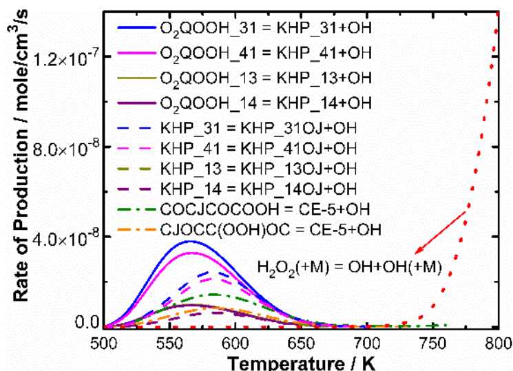
Figure VI. 17 : Prédiction par la modélisation de la production du radical OH par différentes réactions dans l'oxydation du 1,2-DME dans les conditions stœchiométriques à 10atm.
