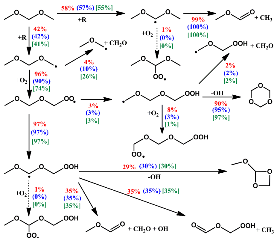
Figure VI. 12 : Voies principales d'oxydation du DMM en JSR à 700 K et 10 atm. Les chiffres indiquent la contribution à la consommation des espèces sources à \phi = 0,2 , 0,5 (parentèses) et 1,5 (crochets).
