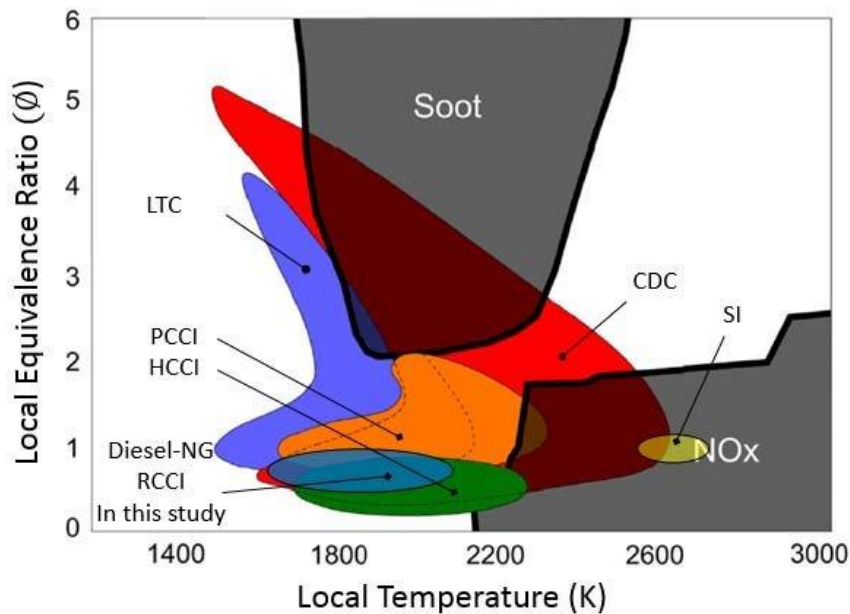
Figure II. 5 : Impact de la richesse et de la température sur les émissions de NOx et de suie [128].
