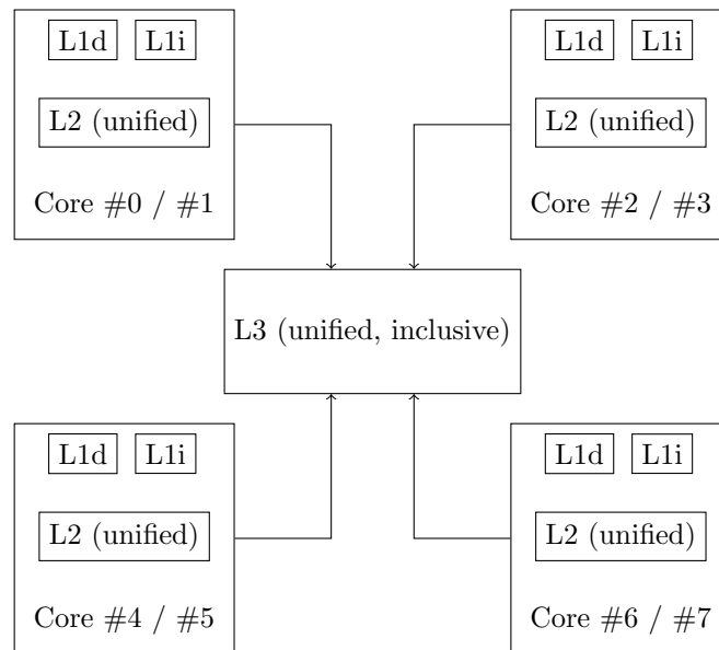
Figure 1: Organisation du cache (exemple)
