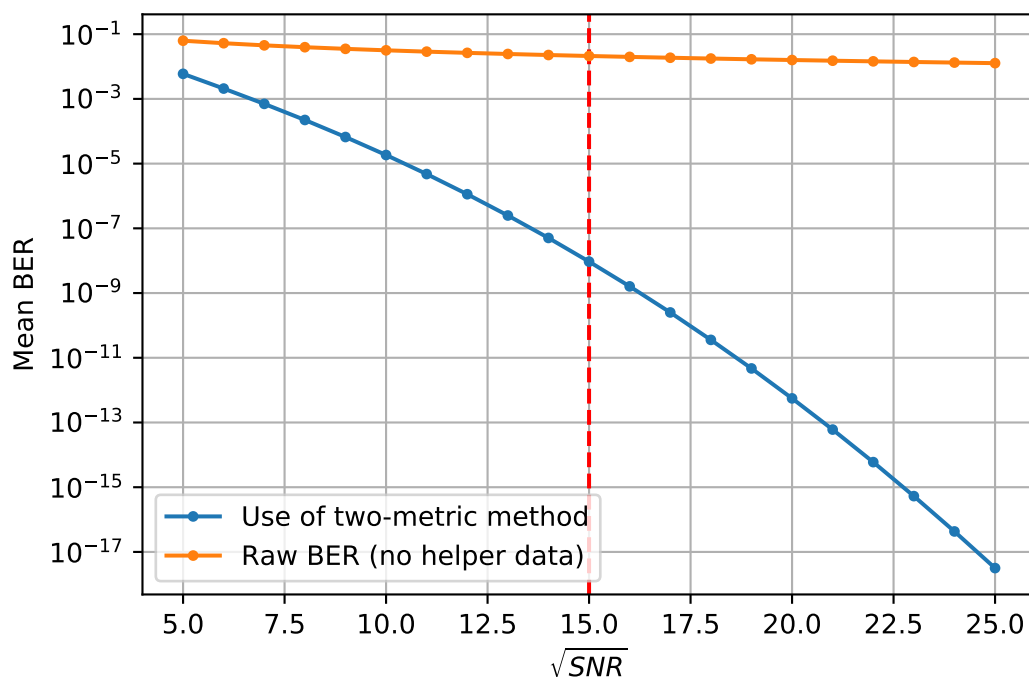
Figure 4: Taux d'erreur binaire en utilisant deux paires de seuils
