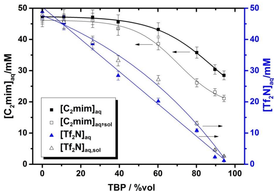
Figure 2-3. Solubilités des ions du LI ( [Tf_2N^-]_{eq,aq} et [C_2mim^+]_{eq,aq} ) en fonction de la concentration en TBP dans la phase organique. Phase aqueuse : LiCl / HCl ( pH_{aq,init} = 2 et [Li^+]_{aq,init} = 15,4 \text{ mmol.L}^{-1} ) ou HCl ( pH_{aq,init} = 2 sans lithium) ; phase organique : TBP / [C_2mim][Tf_2N] .
