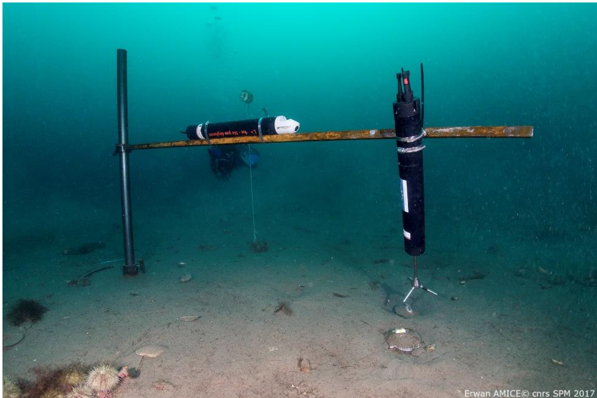
Figure 4 : Photo in situ d'un ADCP et d'un ADV placés au-dessus d'un P. magellanicus équipé d'un accéléromètre (Source : E. Amice/CNRS).
