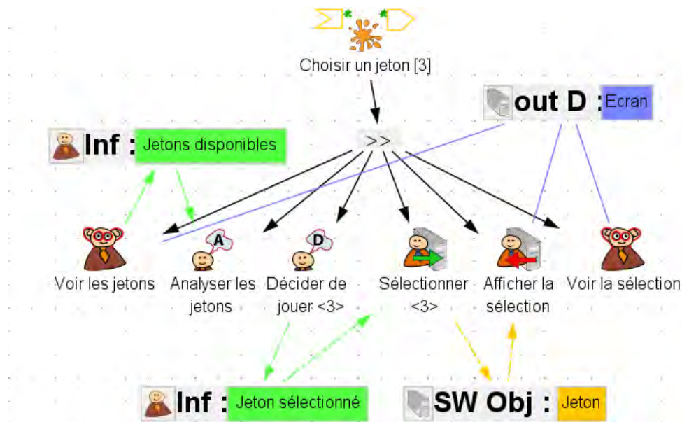
Figure 41. Composant le paramètre "jeton" instancié avec la valeur 3.
