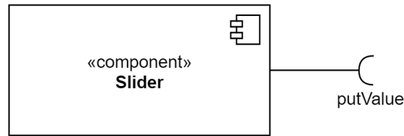
Figure 1.2 – Représentation en UML 2.0 du composant Slider avec un service requis putValue
