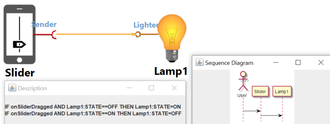
Figure 7.2 – Application d'éclairage ambiant modifiée autrement par l'utilisateur
