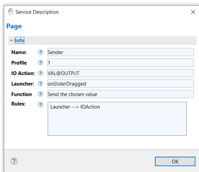
Figure 10.5 – Fenêtre de description d’un service
