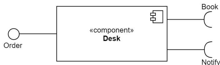
Figure 1.1 – Représentation en UML 2.0 du composant Desk et de ses services
