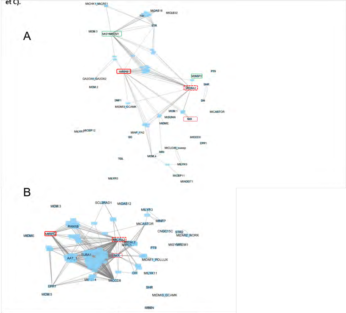
Figure 43 : Sous-réseaux génomiques d'interactions génétiques (au moins trois arêtes par gènes) pour des gènes impliqués dans les symbioses rhizobiennes et mycorhiziennes chez M. truncatula (A, B, C: population entière, FW et C).
