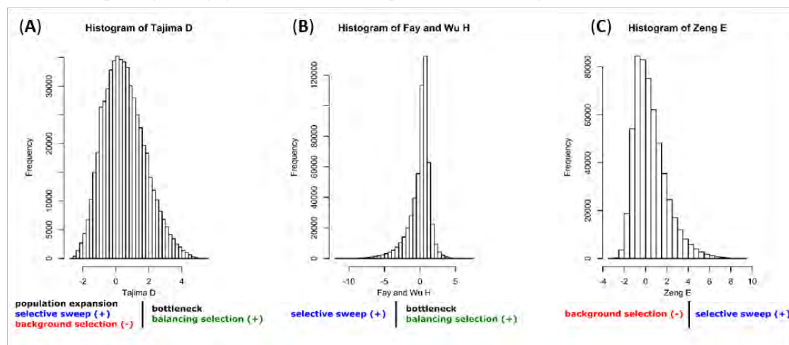
Figure 13 : Distributions théoriques des tests de Neutralité. Distribution du D de Tajima (A), du H de Fay & Wu (B) et du E de Zeng (C). Sous chacune des distributions, il est indiqué comment les différents modes de sélection influencent ces distributions vers des valeurs positives ou négatives. Les forces démographiques de « bottleneck », d'expansion et de structuration génétique des populations influencent également ces statistiques.
