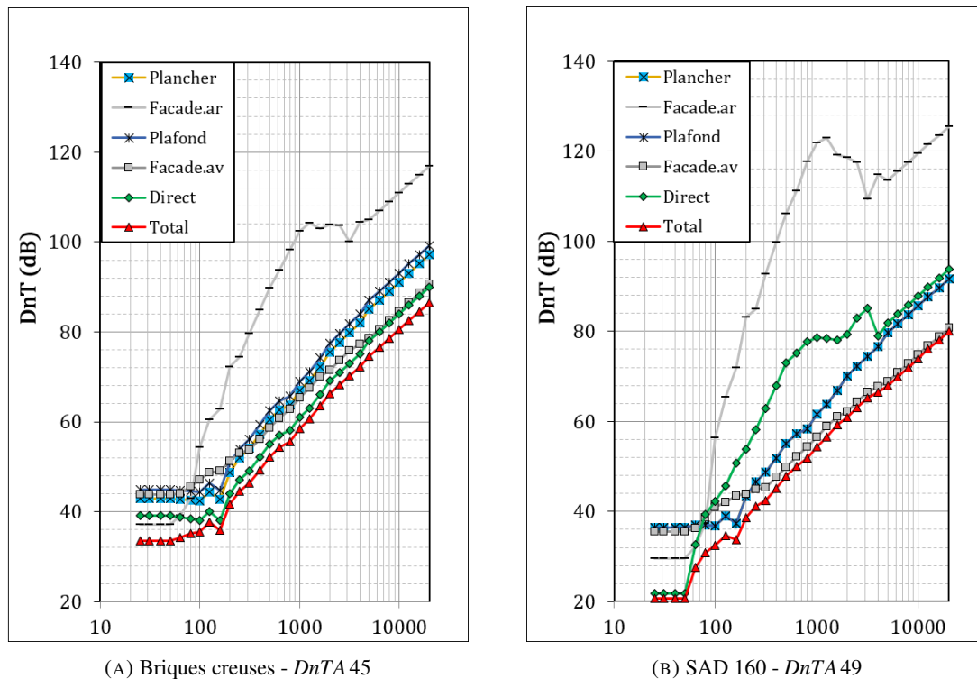
FIGURE 3.19 – Courbes d’isolements in situ par chemin de transmission estimées selon la norme ISO12354-1 2017 pour deux types de séparatifs voisin : (A) Briques creuses ; (B) Cloison SAD160.
