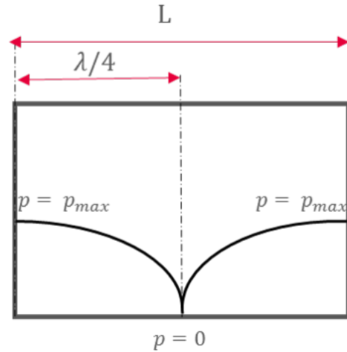
FIGURE 3.12 – Schéma représentant le premier mode d'une salle parallélépipédique aux murs rigides.
