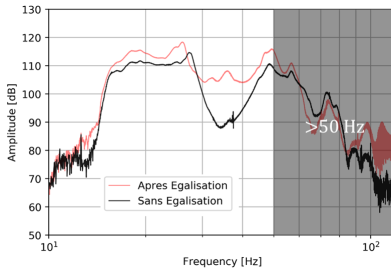
FIGURE 3.13 – Fonction de transfert du caisson de basses Genelec 7070A sans et avec égalisation par filtres en cascades IIR.
