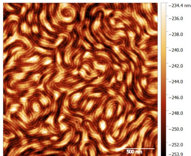
Figure 7 Image de topographie AFM 2 \times 2 \mu\text{m}^2 d'un film de PS- b -P2VP après avoir été plongé dans une solution de tosyle de fer et rincé.
