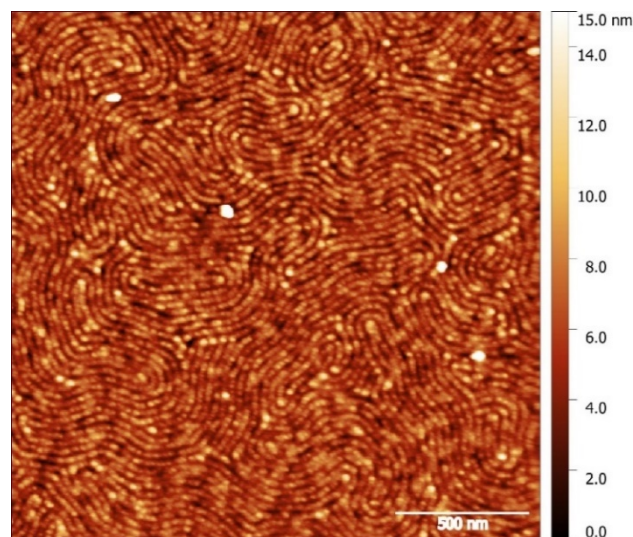
Figure 6 Image de topographie AFM 2x2µm 2 d'un film de PEDOT:Tos après lithographie avec un copolymère à blocs lamellaire.
