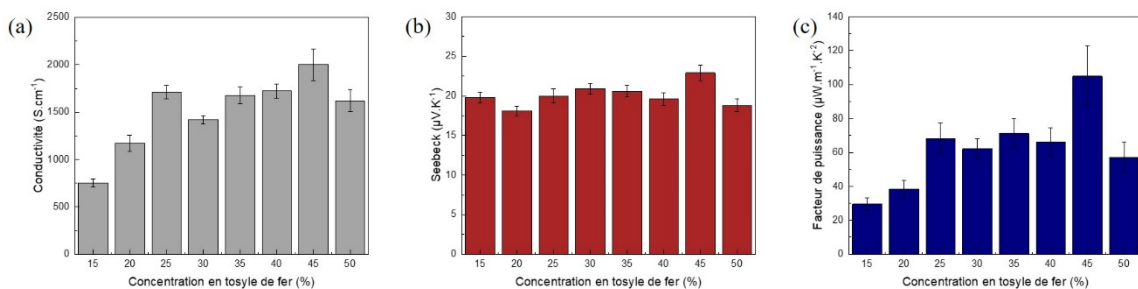
Figure 4 Conductivité électrique, coefficient Seebeck et facteur de puissance des films de PEDOT:Tos en fonction de la concentration en tosylo de fer.
