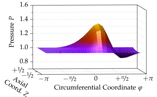
(d) Pressure field ( N_\varphi \times N_Z = 25 \times 5 , N_P = 1 ).
