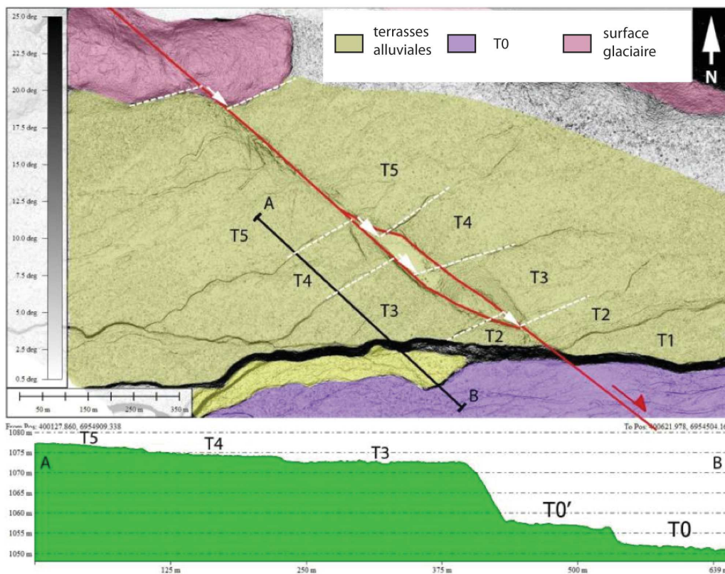
Figure 93 : Terrasses alluviales d'un drain au Sud de la rivière Tetlin, décalées horizontalement (voir localisation sur la Figure 92, rectangle orange). La figure du bas présente une coupe topographique de ces terrasses selon le profil AB extrait du MNT IfDEM (Laurent Bourillon) (carte de pentes MNT IfDEM).
