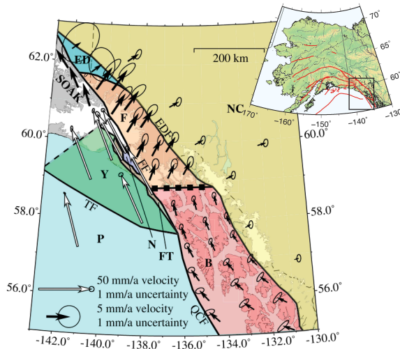
Figure 150 : Modèle de bloc pour la partie Est de la syntaxe, et vitesses calculées par rapport à la plaque Nord-Amérique. Voir texte pour les abréviations des noms de blocs (Elliott et al., 2010).
