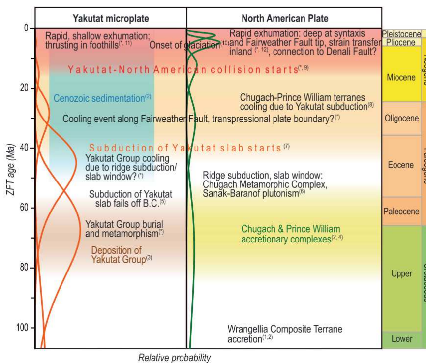
Figure 9 : Résumé graphique des événements tectoniques (Falkowski et al., 2014). La courbe orange correspond aux pics d'exhumation pour la microplaque Yakutat et la courbe verte pour la plaque Nord-Amérique.
