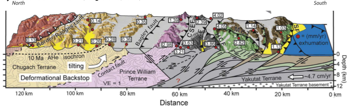
Figure 8 : Coupes schématiques à l'échelle crustale au niveau de l'accrétion du bloc Yakutat dans la syntaxe Est (A) (Chapman et al., 2012) et Centre/Ouest (B) (Berger et al., 2008).
