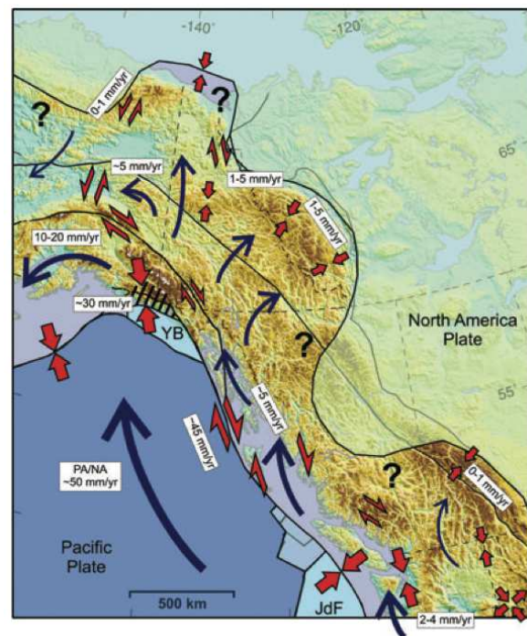
Figure 33 : Tectonique active de la partie Nord de la Cordillère à partir des données de sismicité, mécanismes au foyer et données GPS. Les flèches bleues montrent les mouvements schématiques et les blocs internes à la Cordillère par rapport à la plaque Nord-Américaine. Les flèches rouges indiquent les zones de décrochement et de raccourcissement. La zone hachurée représente la zone de collision Yakutat principale (Mazzotti et al., 2008).
