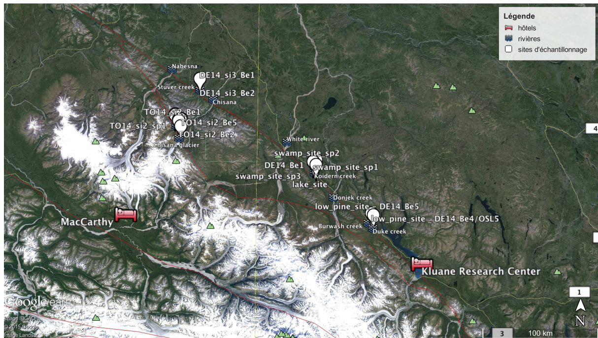
Figure 78 : Localisation des sites d'échantillonnage de la mission en géomorphologie de Septembre 2014.
