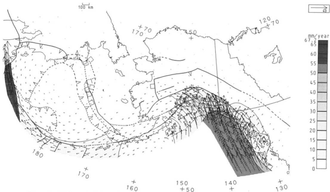
Figure 36 : Vitesses de surface relatives à la plaque Nord Américaine prédites par le modèle numérique (Bird, 1996).
