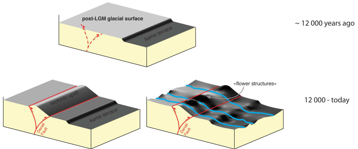
Figure 109 : Blocs diagramme reconstituant la formation des monticules alignés le long de la faille de Denali. Ils sont issus de la combinaison de soulèvement tectonique associé à une structure en pop-up superficielle et de l'érosion de la surface LGM par incision fluviale.
