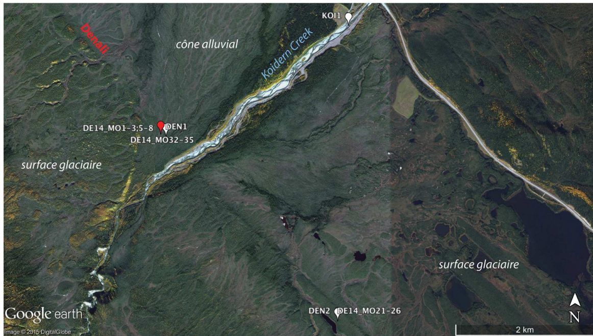
Figure 123 : Echantillons prélevés sur le site Koidern Creek. Les marqueurs blancs indiquent les échantillons de ^{10}\text{Be} , les marqueurs rouges les échantillons de ^{14}\text{C} .
