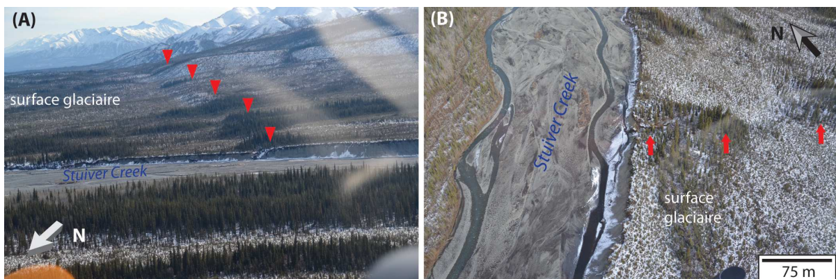
Figure 97 : A : Photographie aérienne de la faille de Denali en rive droite de la Stuver Creek (voir Figure 96 pour la direction indiquée par l'œil). L'escarpement de faille est indiqué par les triangles rouges. B : Photographie aérienne quasi verticale du talus entre la rive droite de la Stuver Creek et la surface glaciaire. La faille est marquée par les flèches rouges : aucun décalage n'est visible au niveau du talus.
