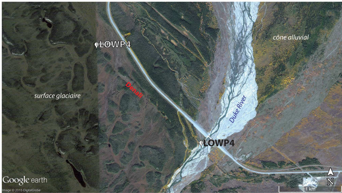
Figure 121 : Echantillons prélevés sur le site Low Pine dans la surface glaciaire (LOWP4) et la rivière Duke (LOWP5).
