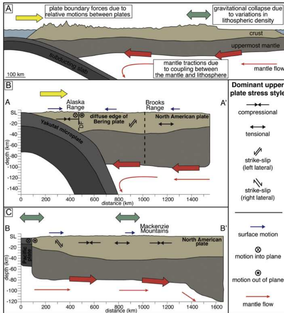
Figure 37 : A : Coupe schématique qui illustre les trois principaux moteurs de la déformation continentale. B-C : Coupes schématiques illustrant la cinématique de surface, l'état de contraintes dominant dans la plaque supérieure et les forces dominantes dans différentes régions (B : coupe NE-SW à travers le Yukon ; C : coupe NO-SE à travers la partie centrale d'Alaska) (Finzel et al., 2014).
