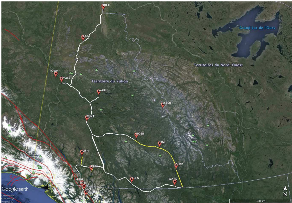
Figure 42 : Stations occupées durant la campagne de mesures de l'été 2013.
