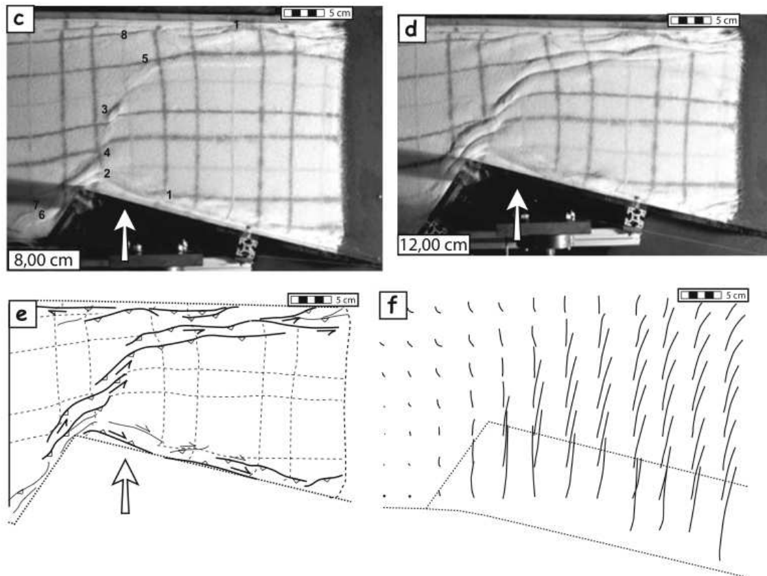
Figure 2 : Modèle analogique d'indenteur pour les Alpes (Rosenberg et al., 2007). Les figures C et D représentent le modèle après 26% et 40% de raccourcissement, respectivement. La figure E montrent les failles majeures de la figure D, et la figure F le flux de particules calculé de 0 à 40% de raccourcissement. La similitude avec la collision Yakutat est marquée (en inversant le système).
