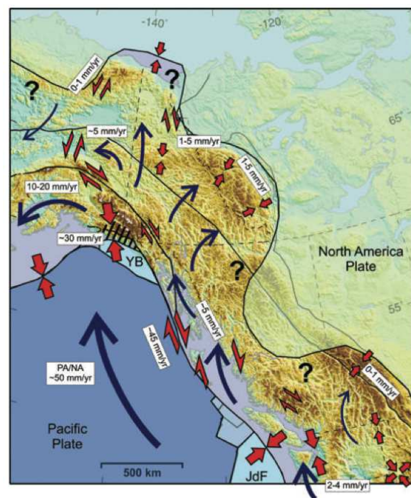
Figure 33 : Tectonique active de la partie Nord de la Cordillère à partir des données de sismicité, mécanismes au foyer et données GPS. Les flèches bleues montrent les mouvements schématisés et les blocs internes à la Cordillère par rapport à la plaque Nord-Américaine. Les flèches rouges indiquent les zones de décrochement et de raccourcissement. La zone hachurée représente la zone de collision Yakutat principale (Mazzotti et al., 2008).
