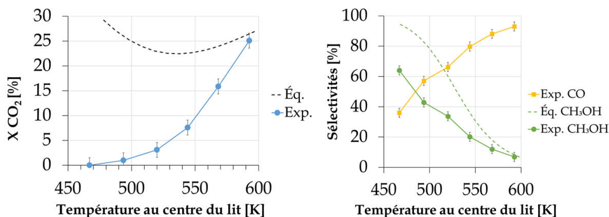
FIGURE 3.12 – Conversion de CO 2 et sélectivité des produits en fonction de la température, catalyseur CuZn/A, 400 mg de catalyseur, d_p = 90 - 200 \mu\text{m} , P = 36 \text{ bar} , N_2/H_2/CO_2 = 4/27/9 , WHSV = 15 \text{ L/g}_{\text{cat}}/\text{h}
