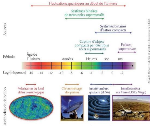
7. Le spectre des ondes gravitationnelles. Il existe de très nombreuses sources attendues d'OG. Différents types de détecteurs ou de méthodes de détection doivent être utilisés selon la bande de fréquence du signal cherché. Les détecteurs interférométriques comme Virgo et LIGO sont des instruments à large bande, sensibles entre quelques dizaines de Hz et 10 kHz.
