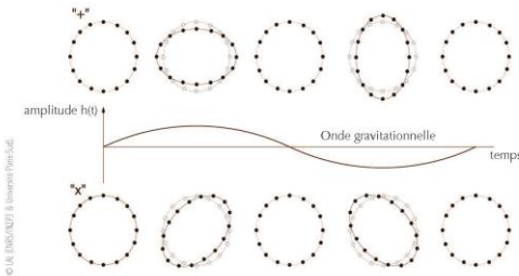
1. Visualisation de l'effet des deux polarisations « + » et « × » d'une onde gravitationnelle sur l'espace-temps. On suppose l'OG périodique et se propageant perpendiculairement au plan de l'image. Un anneau de particules test initialement rond est déformé et se transforme en une ellipse : les longueurs se contractent et s'étirent alternativement dans deux directions perpendiculaires lors du passage de l'OG.
