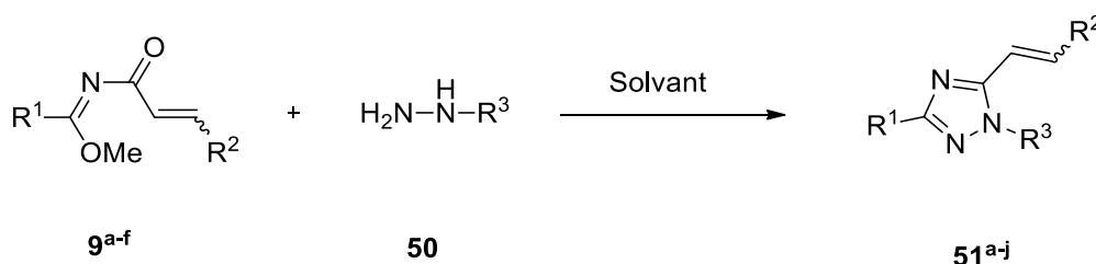
Schéma I.21 : Synthèse des 5-Alcényl-1,2,4- triazoles
