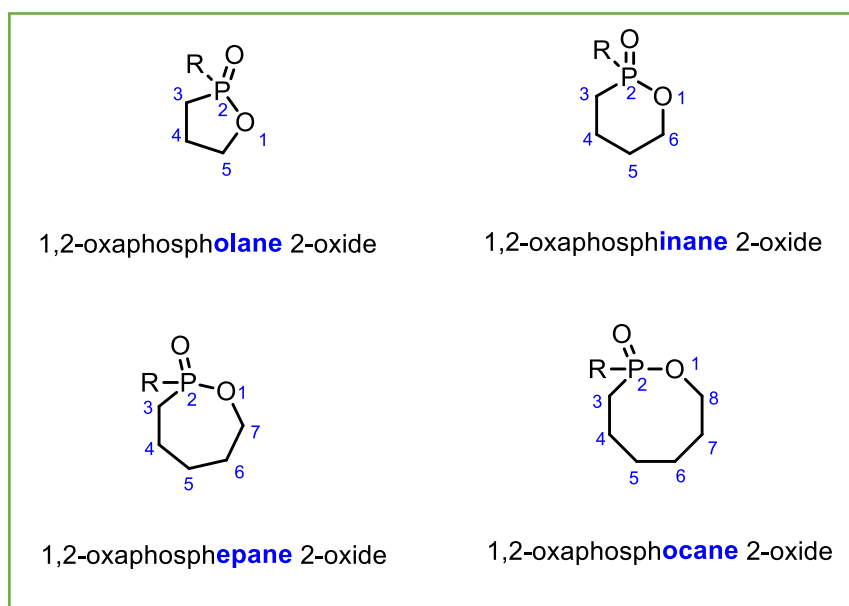
Figure III. 4. Nomenclature des O-P-hétérocycles
