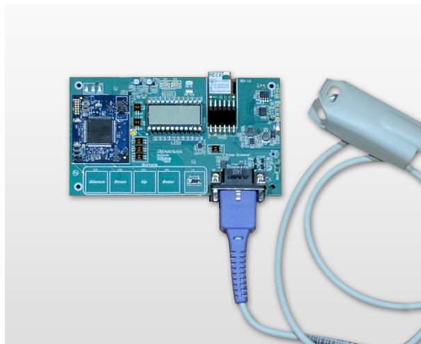
FIGURE 4.3 – Module oxymètre de pouls RENESAS .
