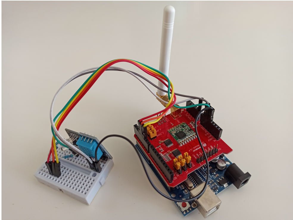
FIGURE 4.7 – Module Dragino LoRa monté sur un Arduino Uno .
