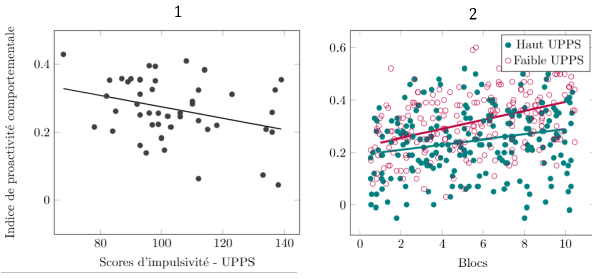
Figure B : (1) Corrélacion entre les scores de personnalité impulsive UPPS et l'indice de proactivité comportementale. (2) Évolution de l'indice de proactivité comportementale au cours des blocs dans le groupe Faible UPPS (ligne et ronds roses, scores inférieurs à la médiane de la distribution) et le groupe Haut UPPS (ligne et ronds verts, scores supérieurs à la médiane de la distribution).
