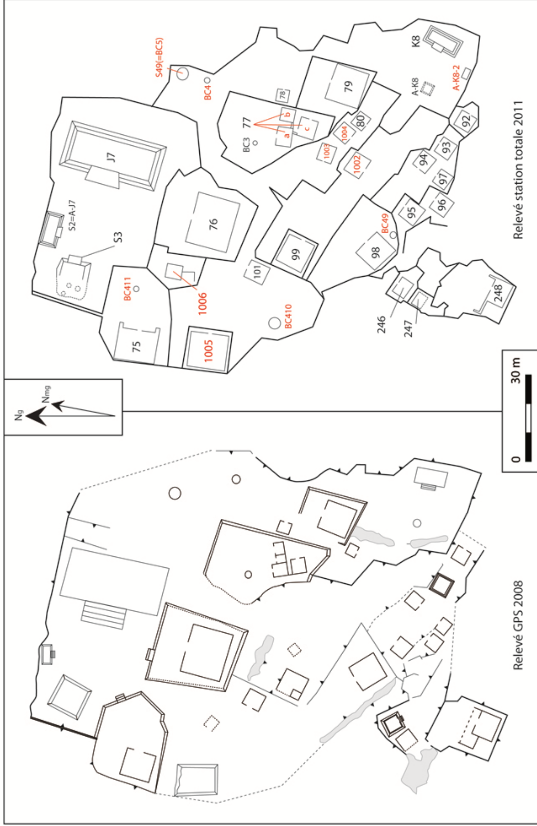
Figure 31 : Comparaison des relevés planimétriques du secteur cérémoniel correspondant aux soubassements pyramidaux J7 et K8 de Malpaïs Prieto.
