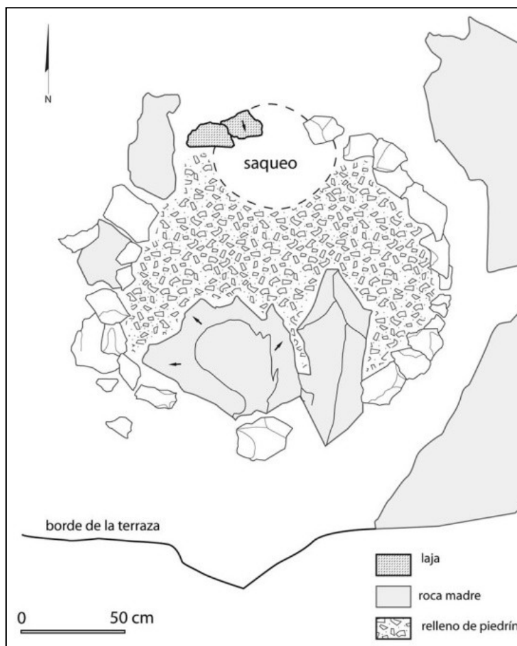
Figure 100 : Relevé en plan de la structure BC407.
