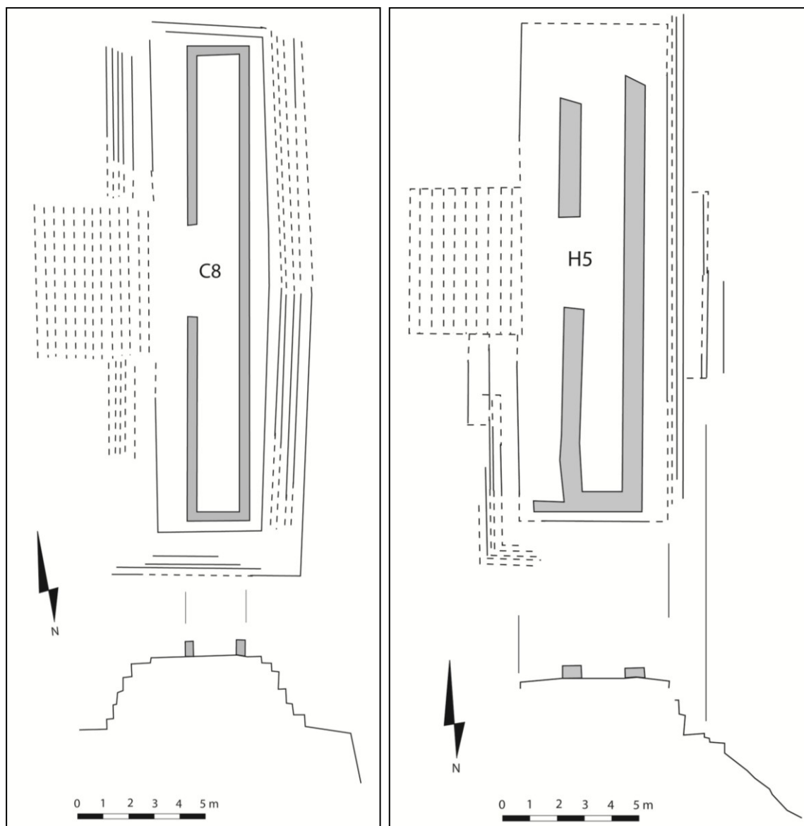
Figure 89 : Relevés en plan des yácatas C8 et H5 de Malpaís Prieto (d'après Michelet 2000).
