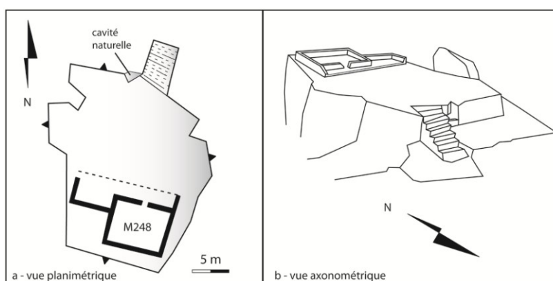
Figure 134 : restitution en plan (a) et en axonomie (b) de la plate-forme de M248.
