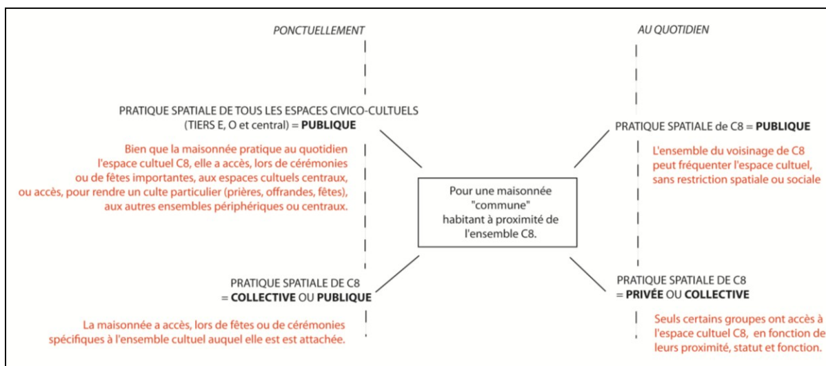
Figure 139 : Schéma récapitulatif des différentes hypothèses relatives à la fréquentation des ensembles cultuels périphériques (exemple de C8).
