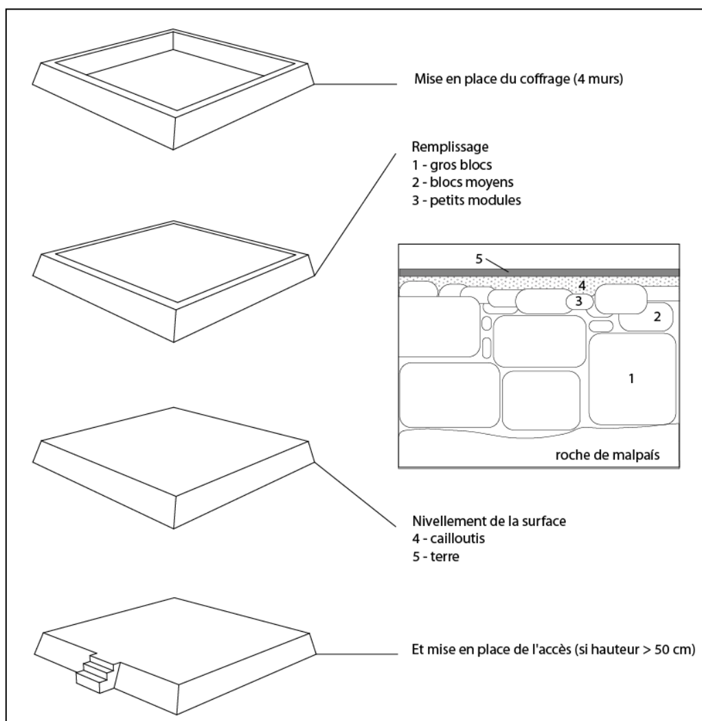
Figure 54 : Détail du système constructif des plates-formes de soubassements « en positif ». Le procédé est identique pour les terrasses, mais est adapté aux irrégularités du terrain.
