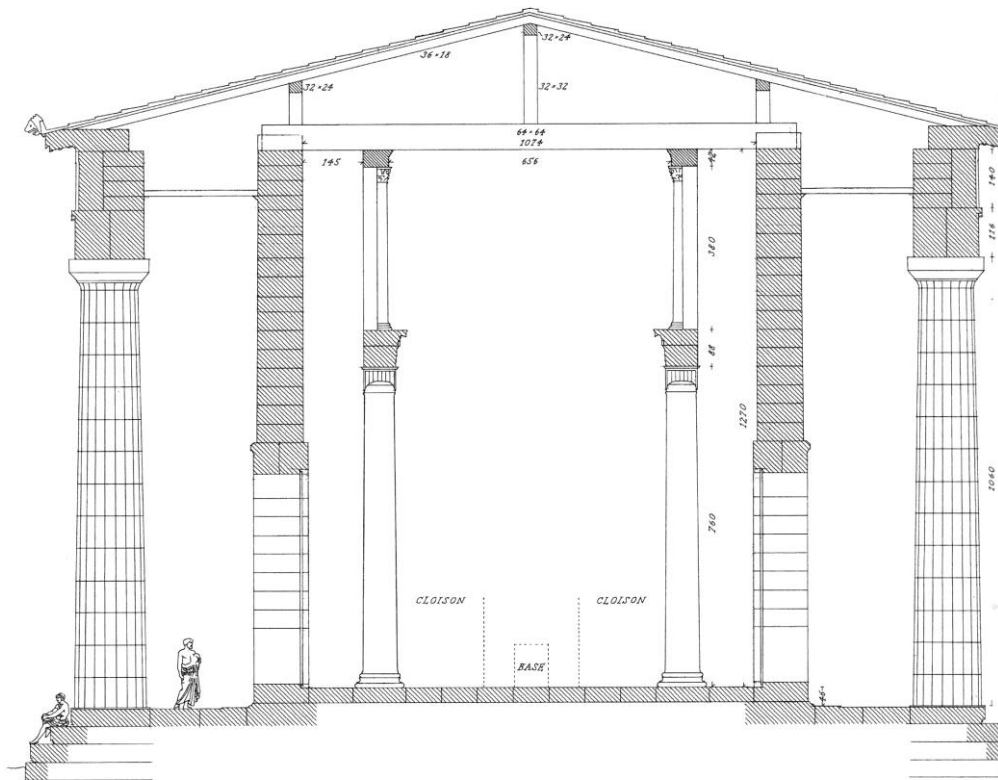
Fig. 18.5. Coupe sur la cella, avec les portes latérales. Essai de restitution éch. 1/125. Les détails des colonnades intérieures sont hypothétiques et la restitution de la charpente est fondée essentiellement sur des calculs de statique. Les mesures sont exprimées en cm.
