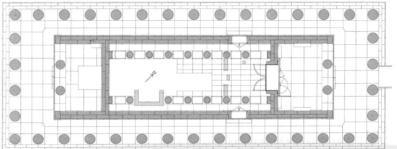
Fig. 18.19. Plan. Restitution éch. 1/225.
