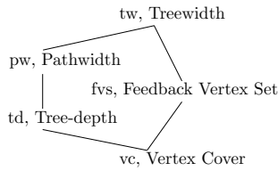
Figure 7.2: Relations entre les paramètres considérés. Les résultats algorithmiques sont hérités à la baisse (de tw à vc ), de la difficulté à la hausse.
