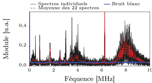
FIGURE 3.1 – Bruit électronique
