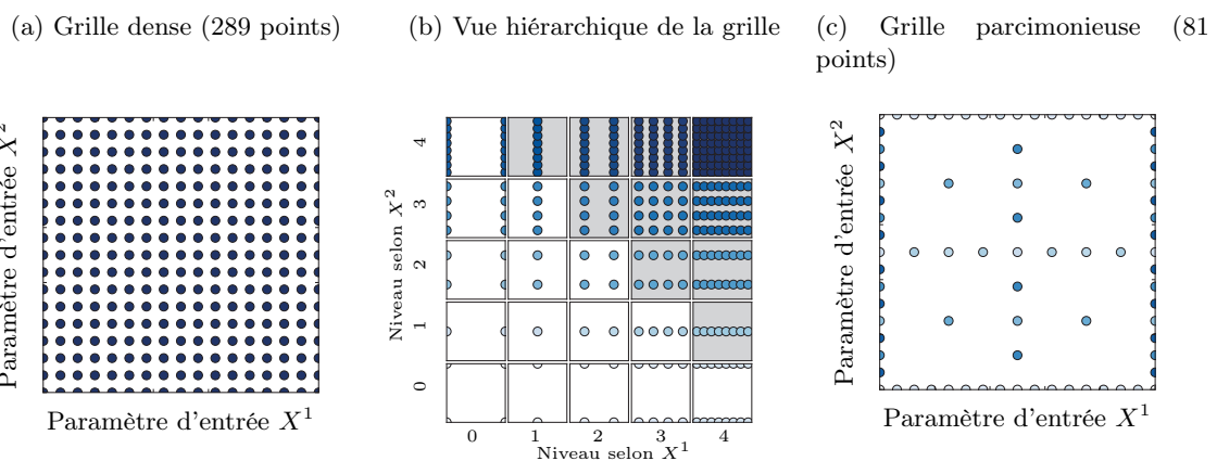
FIGURE 2.12 – Construction d'une grille parcimonieuse pour deux paramètres d'entrée Une grille dense consiste à échantillonner régulièrement les paramètres d'entrée puis à observer la sortie du méta-modèle pour toutes les combinaisons possibles de ces entrées. La grille hiérarchique réorganise la grille dense en une superposition de grilles de plus en plus fines. Sur la vue hiérarchique 2.12b, les grilles à fond gris montrent une densité de points supérieure à celle des autres grilles, si bien que l'information portée par chacun de ces points n'est utile que sur un domaine limité : en les supprimant, une grille parcimonieuse est obtenue.
