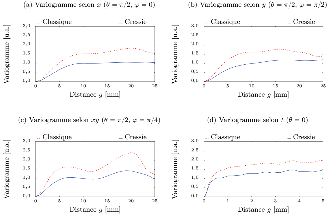
FIGURE 3.8 – Variogramme calculé sur la texture de la Figure 3.5
