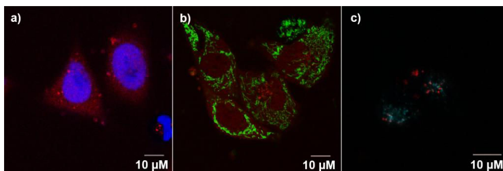
Figure 71. Images confocales de cellules HeLa après 24h d'incubation avec \text{P}(\text{GdDTTA})_4 (1 \mu\text{M} ). Fluorescence de \text{P}(\text{GdDTTA})_4 en rouge, a) Hoescht (bleu), b) mitotracker (vert) et c) lysotracker (cyan).
