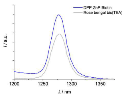
Figure 106. Luminescence de l'oxygène singulet produit dans le DCM suite à l'excitation du PS DPP-ZnP-Biotine et la référence, le Rose Bengal.
