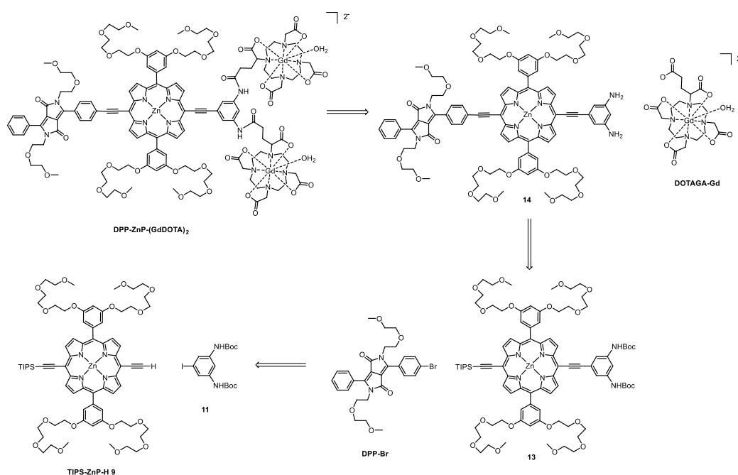
Figure 40. Rétrosynthèse de DPP-ZnP-(GdDOTA) 2 .
