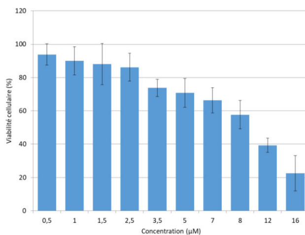
Figure 81. Viabilité cellulaire après 24 h d'incubation avec GdDOTA-ZnP-ZnP-GdDOTA de cellules HeLa. ( C_{\text{mère}} = 10^{-3} M dans le DMSO).
