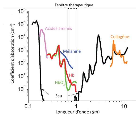
Figure 5. Absorbance de différents composés endogènes pour des longueurs d'onde allant de 200 à 10000 nm. Image adaptée avec autorisation du journal. 36
