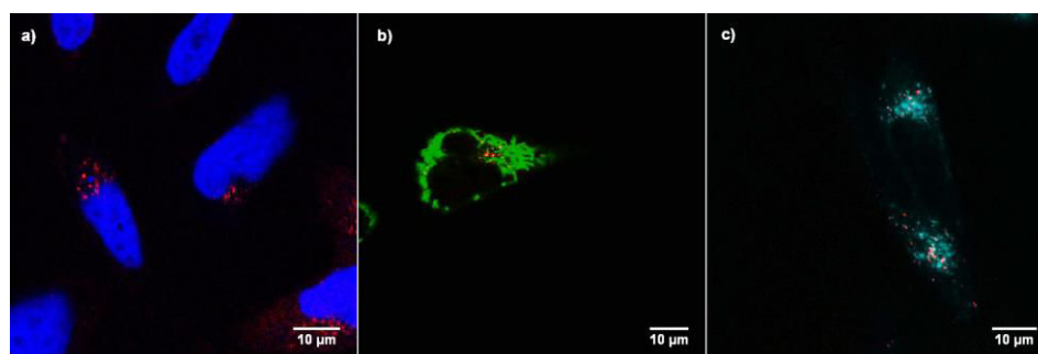
Figure 79. Images confocales de cellules HeLa après 24h d'incubation avec GdDOTA-ZnP-ZnP-GdDOTA (1 \mu\text{M} ). GdDOTA-ZnP-ZnP-GdDOTA en rouge , a) Hoescht (bleu), b) mitotracker (vert) et c) lysotracker (cyan).
