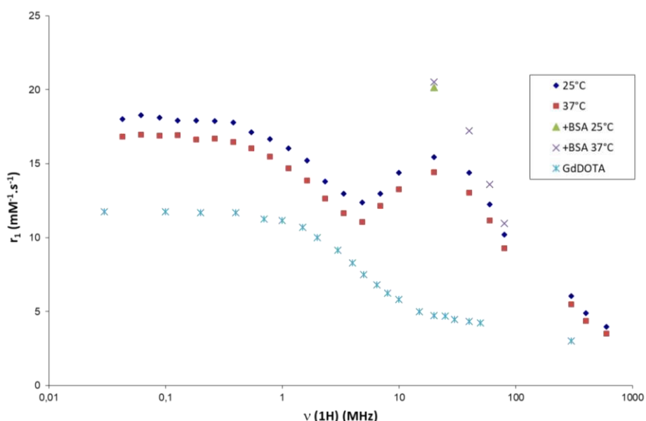
Figure 62. Profil NMRD de DPP-ZnP-(GdDOTA) 2 (1,02 mM dans H 2 O/1 % DMSO, pH = 7,3) et GdDOTA (eau, pH = 5,1, 25 °C).
