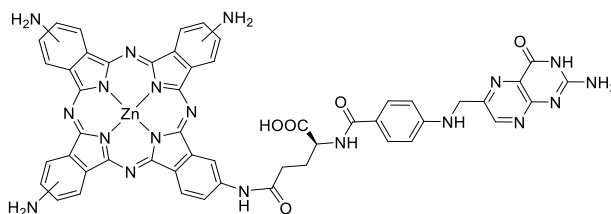
Figure 34. Structure de la phthalocyanine de zinc(II) reliée à l'acide folique par Chen et al .
