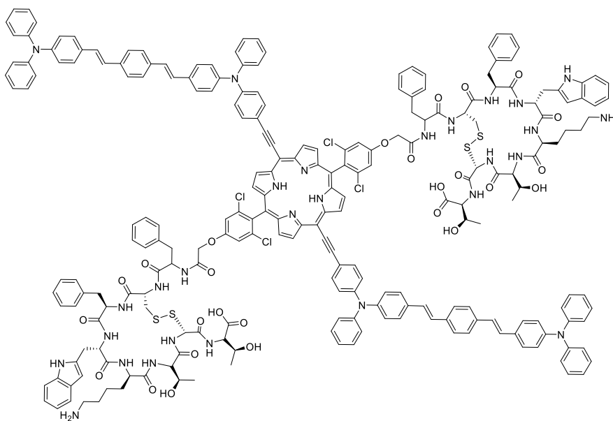
Figure 33. Structure du PS pour la PDT par excitation biphotonique vectorisé décrit par Spangler et al .
