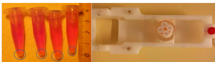
Figure 74. A gauche : eppendorfs contenant les culots cellulaires. A droite : eppendorfs placés dans le dispositif allant dans l'appareil IRM (7 T).
