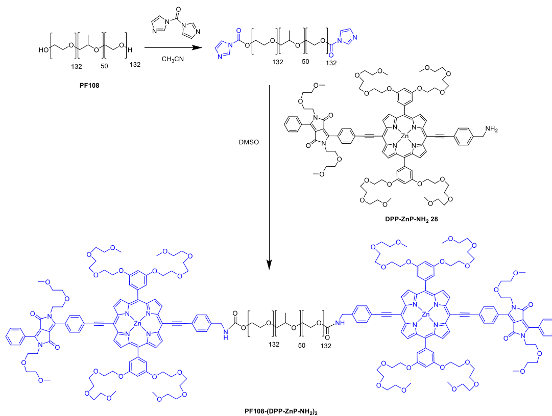
Figure 127. Schéma de synthèse de PF108-(DPP-ZnP-NH 2 ) 2 .
