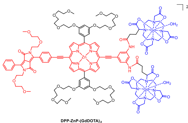
Figure 35. Structure du composé DPP-ZnP-(GdDOTA) 2 .
