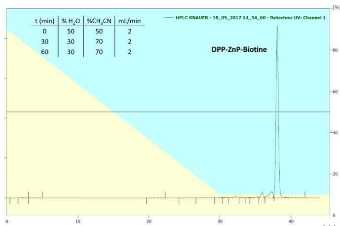
Figure 98. Chromatogramme HPLC de DPP-ZnP-Biotine et le gradient d'élution.
