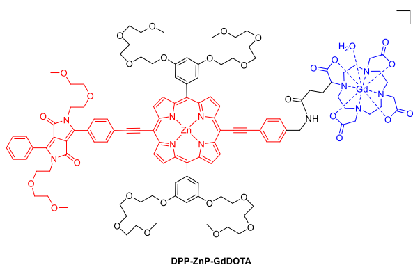
Figure 39. Structure du composé théranostique DPP-ZnP-GdDOTA .
