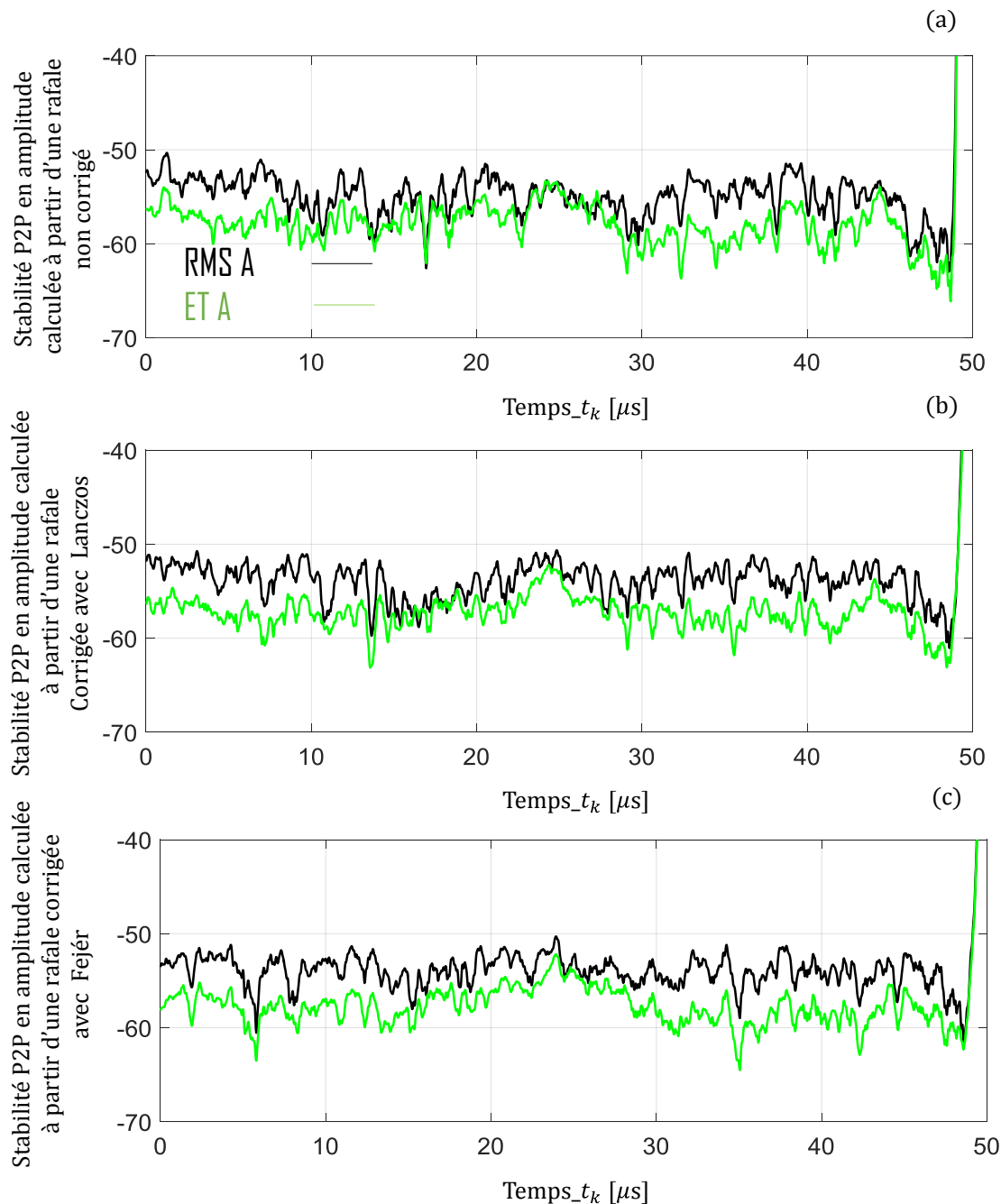
Figure III. 27: Superposition des deux stabilités P2P en amplitude calculées sur les six dernières impulsions avec les méthodes RMS/ET pour les trois types de rafales : (a) : non-corrigée, (b) :corrignée avec Lanczos et (c) :corrignée avec Fejér avec \tau = 50\mu s, N = 8, tm = td = 13ns .
