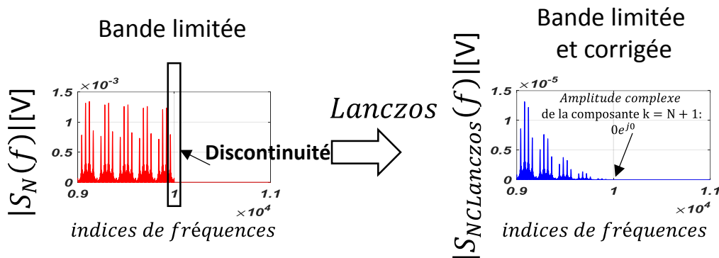
Figure I. 30: Spectres d'un signal rectangulaire limité à la N^{\text{ième}} composante et corrigé autour de la N^{\text{ième}} composante en utilisant les facteurs de Lanczos [19].
