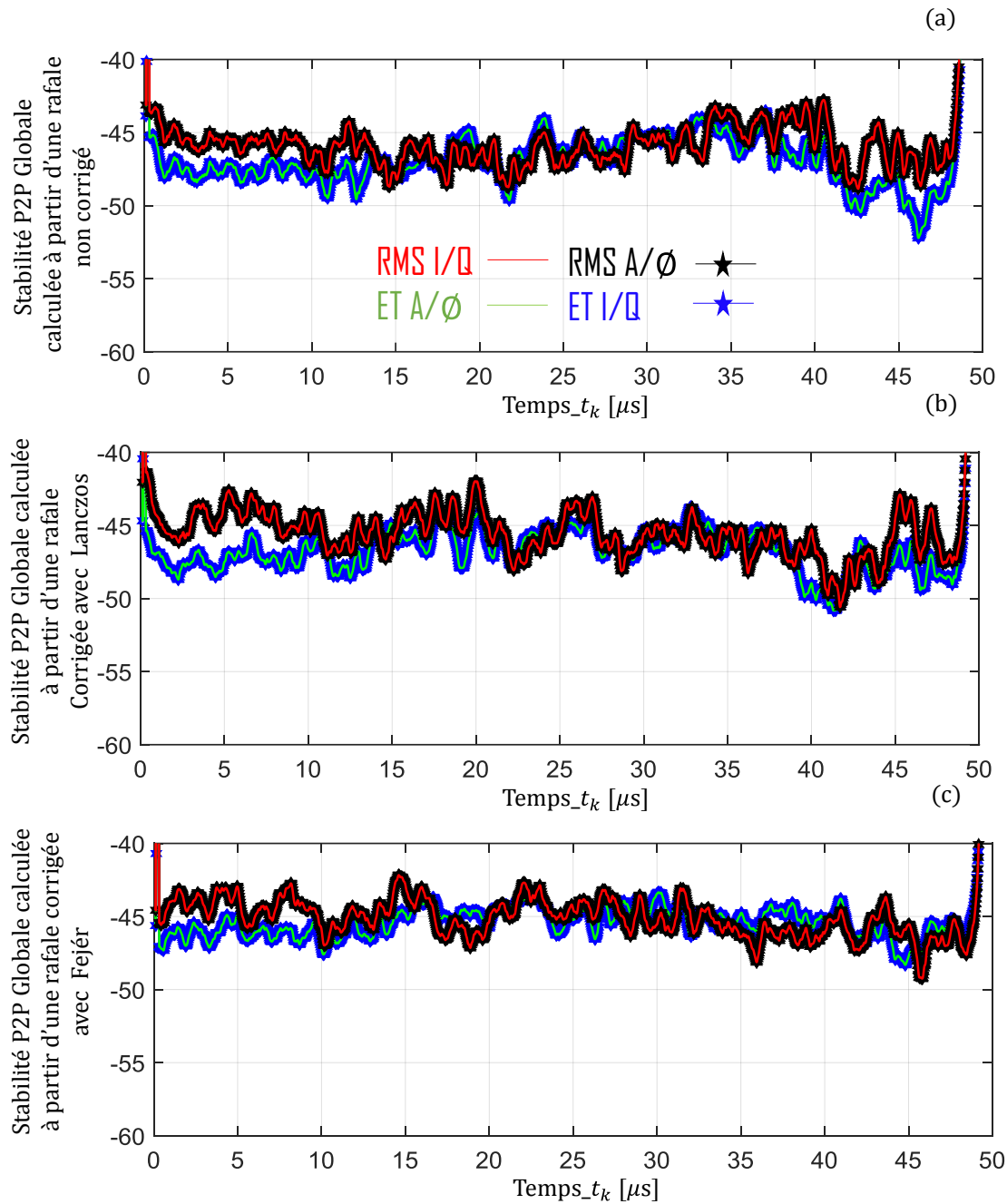
Figure III. 17: Superposition des quatre stabilités P2P en amplitude/phase et en partie réelle/imaginaire calculées avec les méthodes RMS/ET pour les trois types de rafales : (a) : non-correctée, (b) : corrigée avec Lanczos et (c) : corrigée avec Fejér pour t_m = t_d = 1\mu s .
