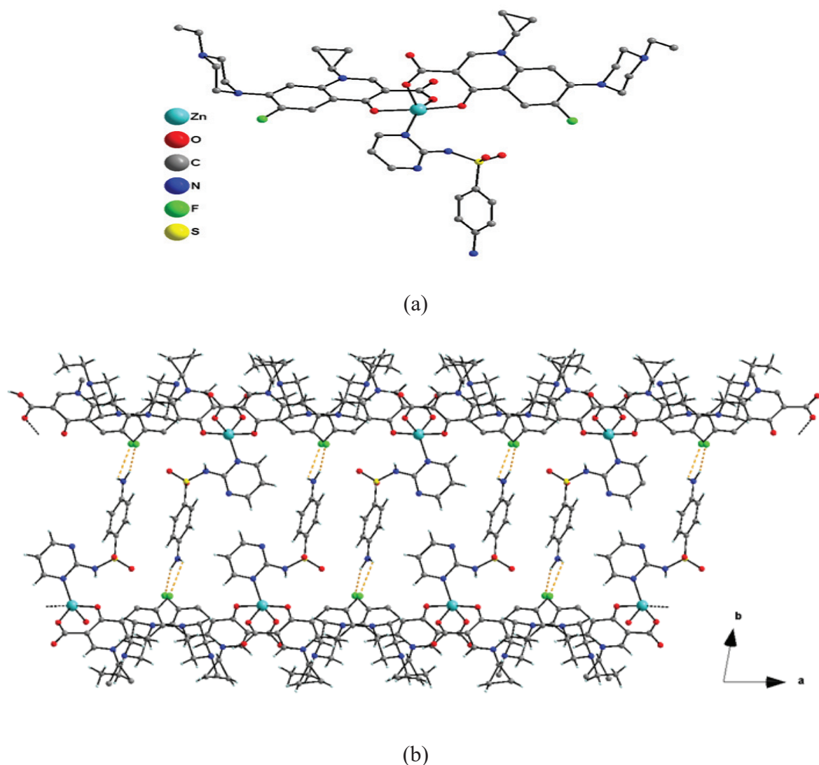
Figure III 28 : (a) Complexe cationique [\text{Zn}(\text{Q1})_2(\text{L1H}_2)]^{+1}, \text{ClO}_4^- . Pour plus de clarté, les atomes d'hydrogène ont été enlevés; (b) Illustration des interactions F...H (lignes pointillées orange) générant des chaînes de complexes courant le long de l'axe a de la cellule unitaire. La présence d'interactions F...H (respectivement entre les ligands Q1H et HL1) génère la formation de pseudo-chaînes de complexes se déplaçant le long de l'axe a de la cellule unitaire (figure III 28b).
