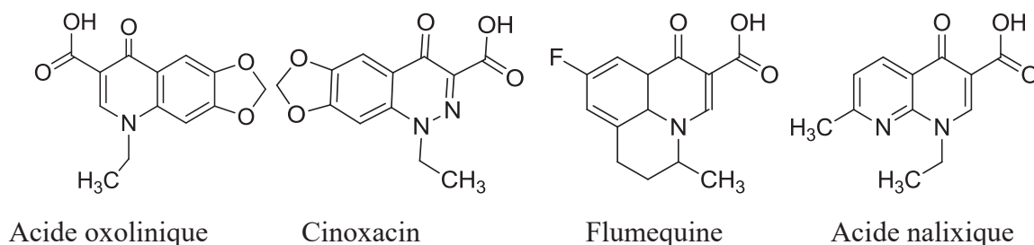
Figure 19 : Les quinolones de la première génération
