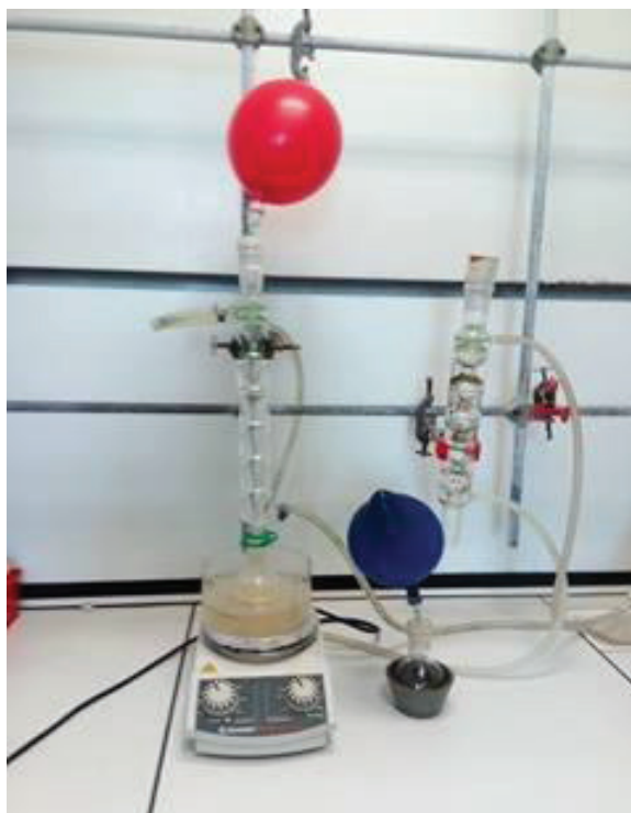
Figure IV 3 : Réaction de condensation d'une sulfonamide
