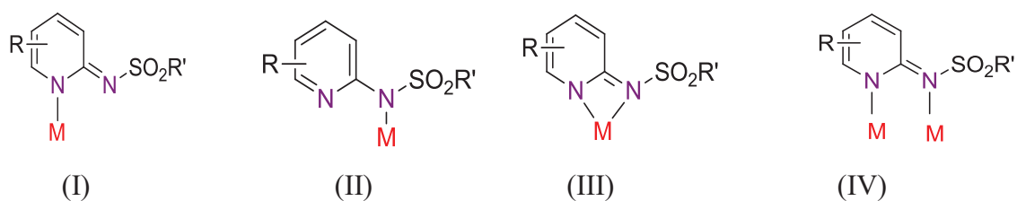
Schéma II : Modes de coordination des sulfamides M: ion métallique. R, R' = alkyle
