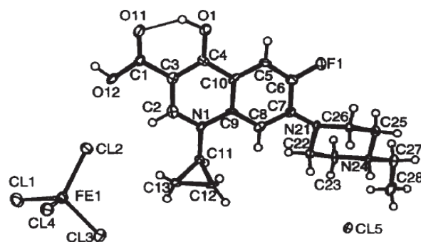
Figure I19 : (erxH_2)[FeCl_4]Cl^{60}
