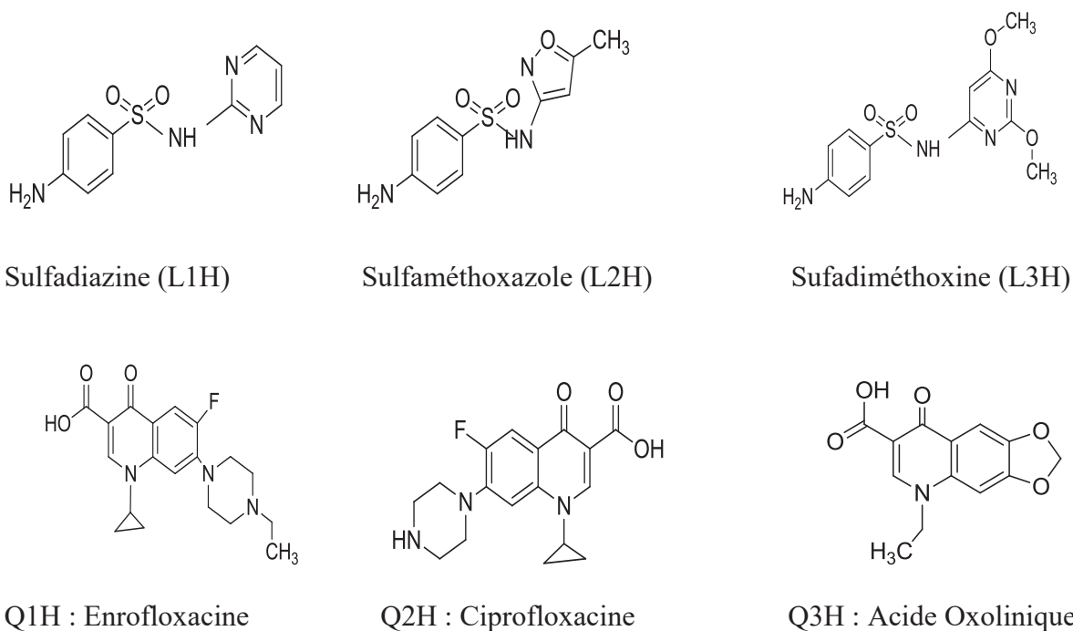
Figure III 20 : Les différents ligands type sulfamides, quinolones utilisés lors de ce travail
