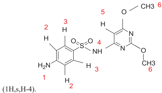
Figure IV 7 : Structure de la sulfaméthoxine non modifiée
